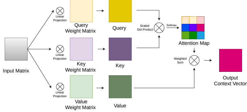
图 3-4 注意力机制通过查询、键和值计算相关性权重并突出关键语音片段
