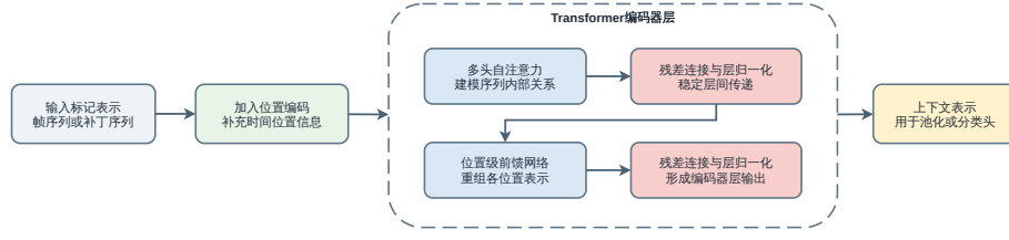
图 3-7 Transformer 编码器层的基本信息流动
