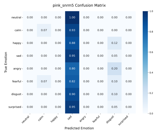
(b) pink 噪声-5dB 条件下的混淆矩阵
