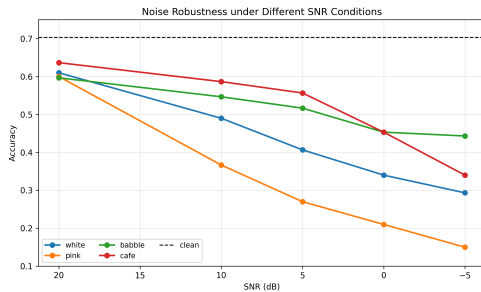
(a) 不同噪声强度下的 Accuracy 变化
