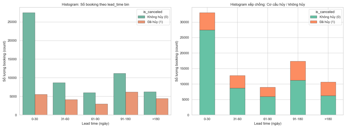
Biểu 1: Histogram số booking theo lead_time bin (tách theo is_canceled)
