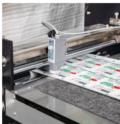
Sistema de detención de alinamiento
