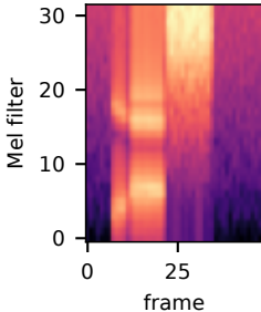
log Mel energy: 32 x 49
