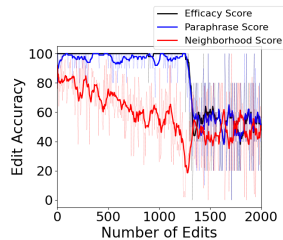
MEMIT on GPT-J.
