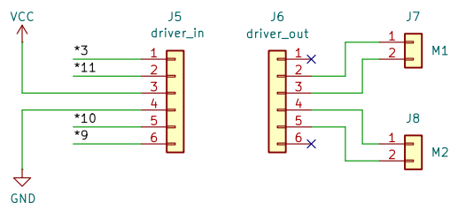
DRIVER DE MOTORES (DRV8833)
