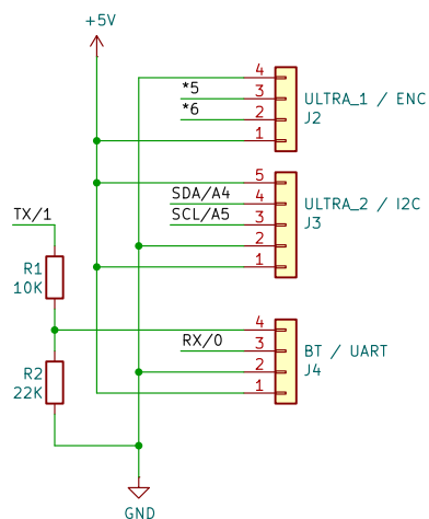
Sensores digitales, BT, I2C
