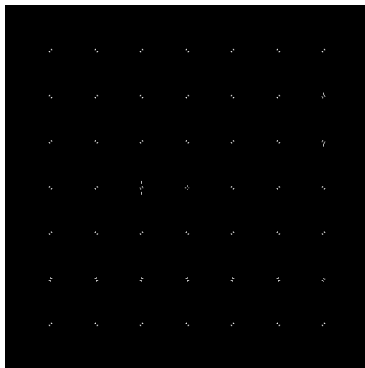
Scharr - b.1
