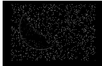
Scharr - b.2
