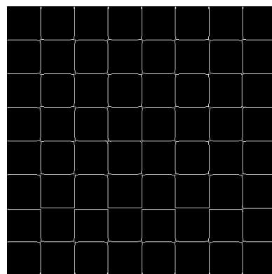
Canny (sigma=1.0)
