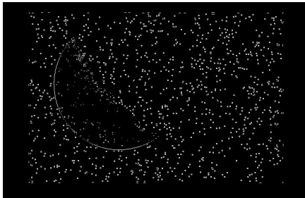
Scharr - b.1
