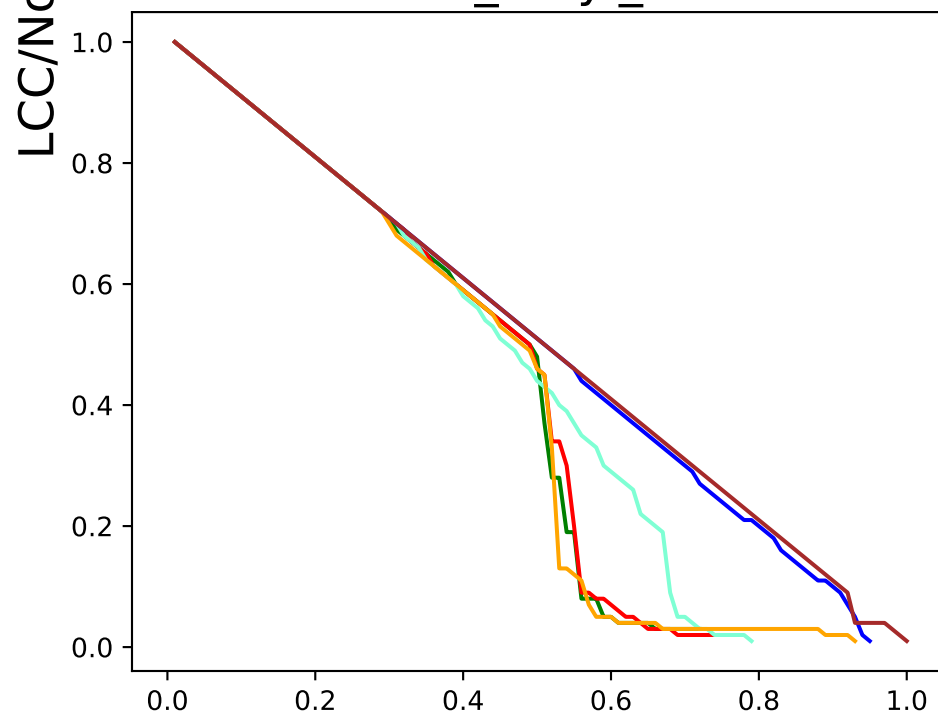
erdos_renyi_100
