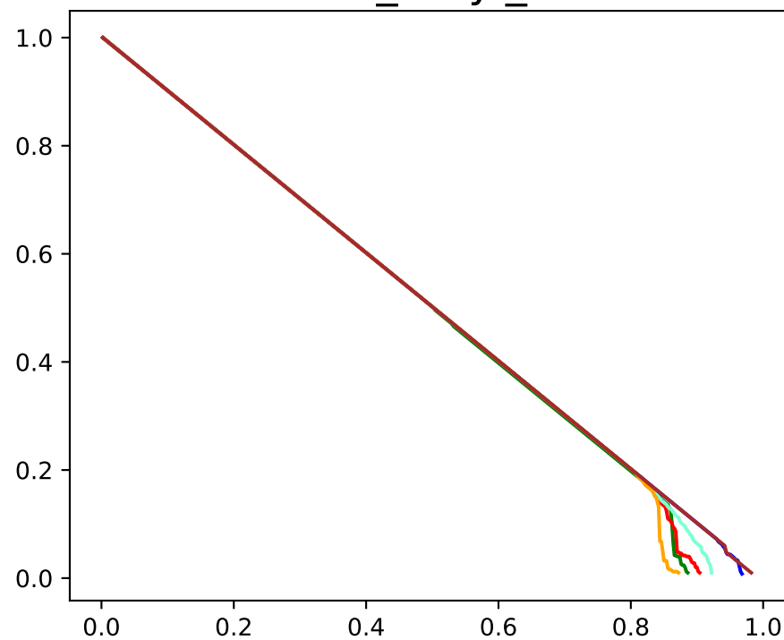
erdos_renyi_500
