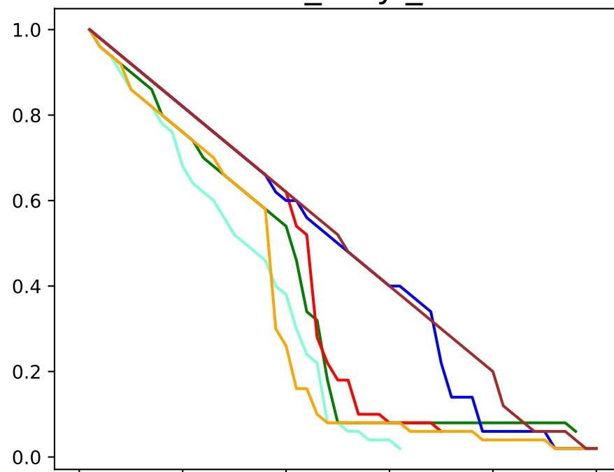
erdos_renyi_50
