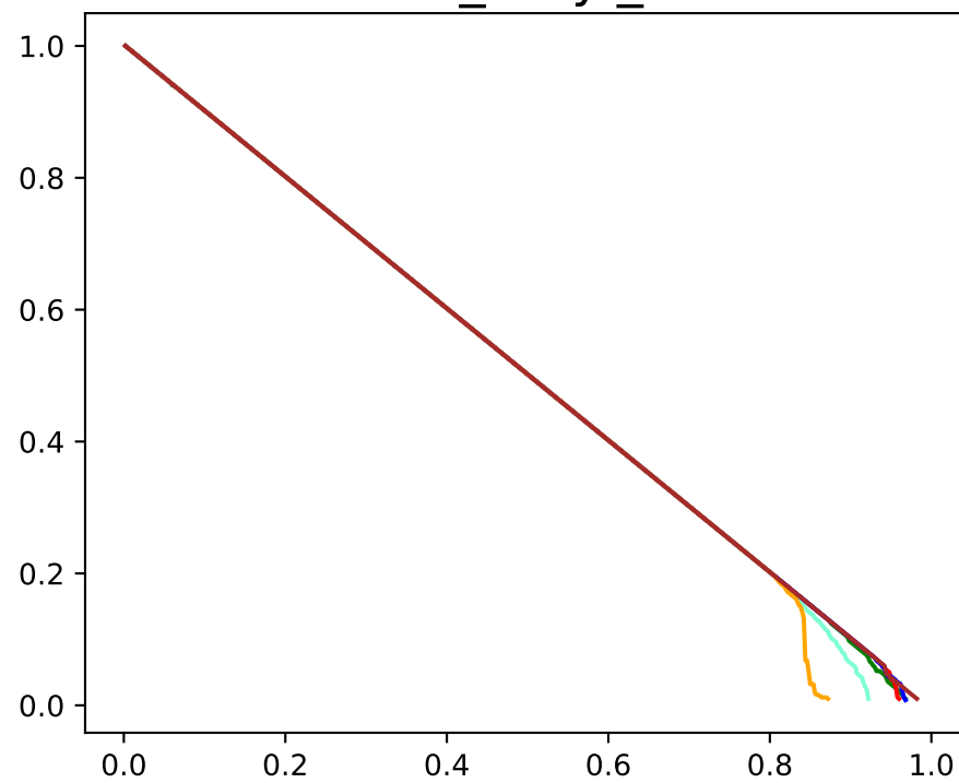
erdos_renyi_500
