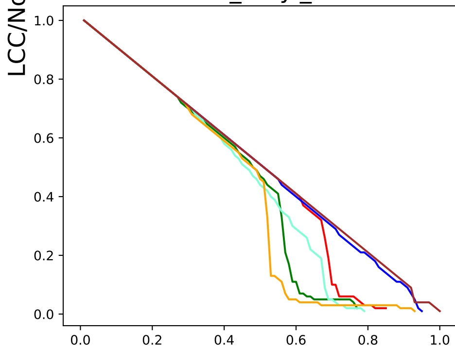
erdos_renyi_100
