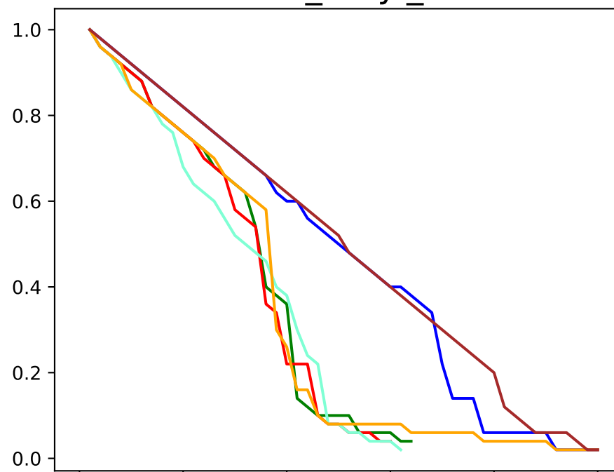
erdos_renyi_50
