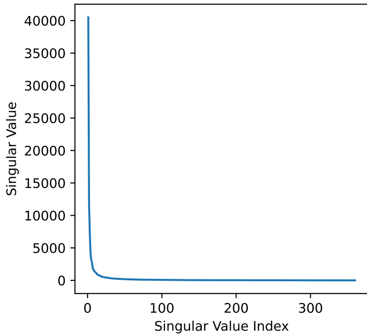
Singular Values
