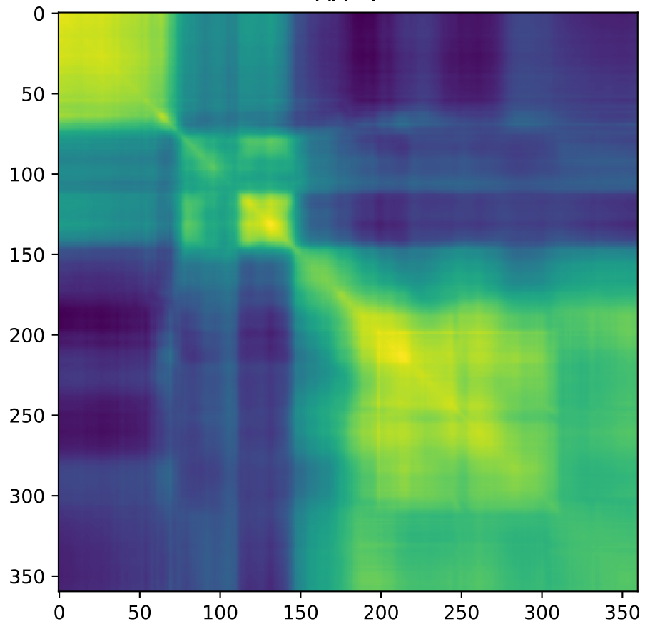
AA^T
