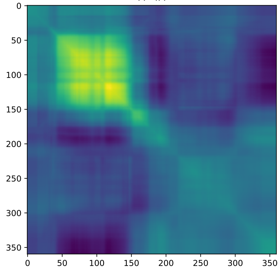
A^T A
