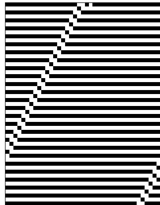
00010001
