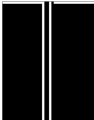
Rule 221
