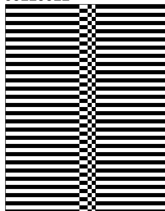
00110011
