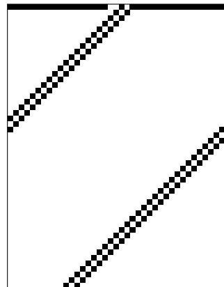
00100010
