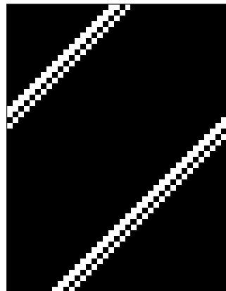
10101010
