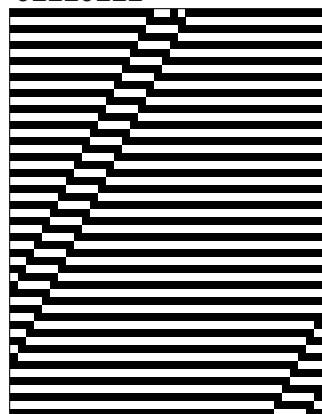
01110111
