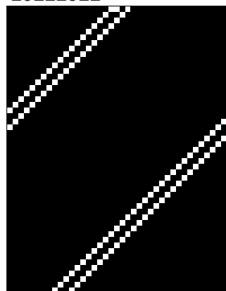
10111011
