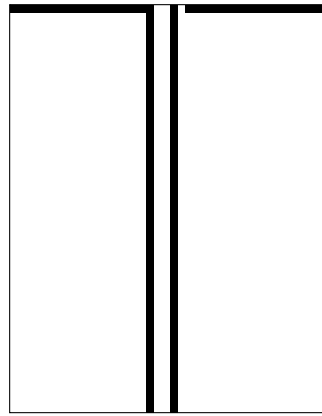
01000100
