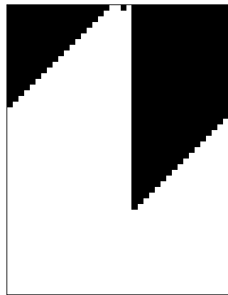
10001000
