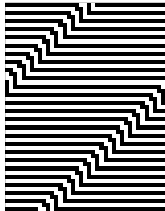
01010101
