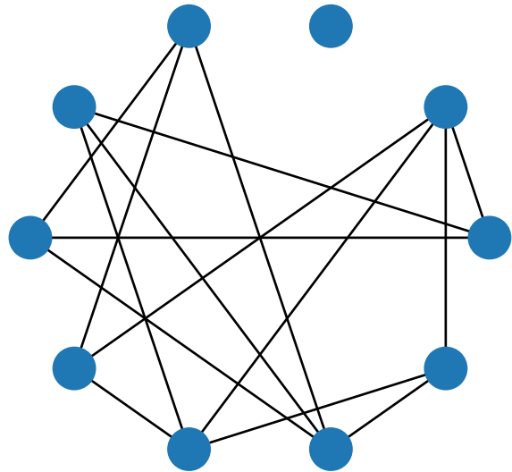
Erdős-Rényi
