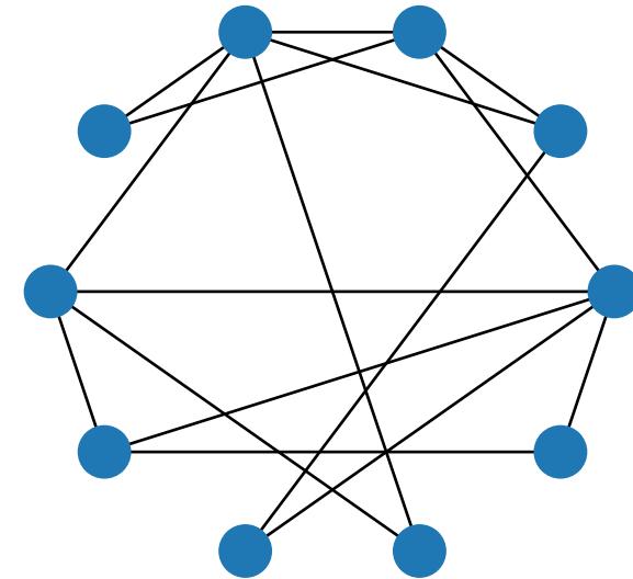
Barabási-Albert
