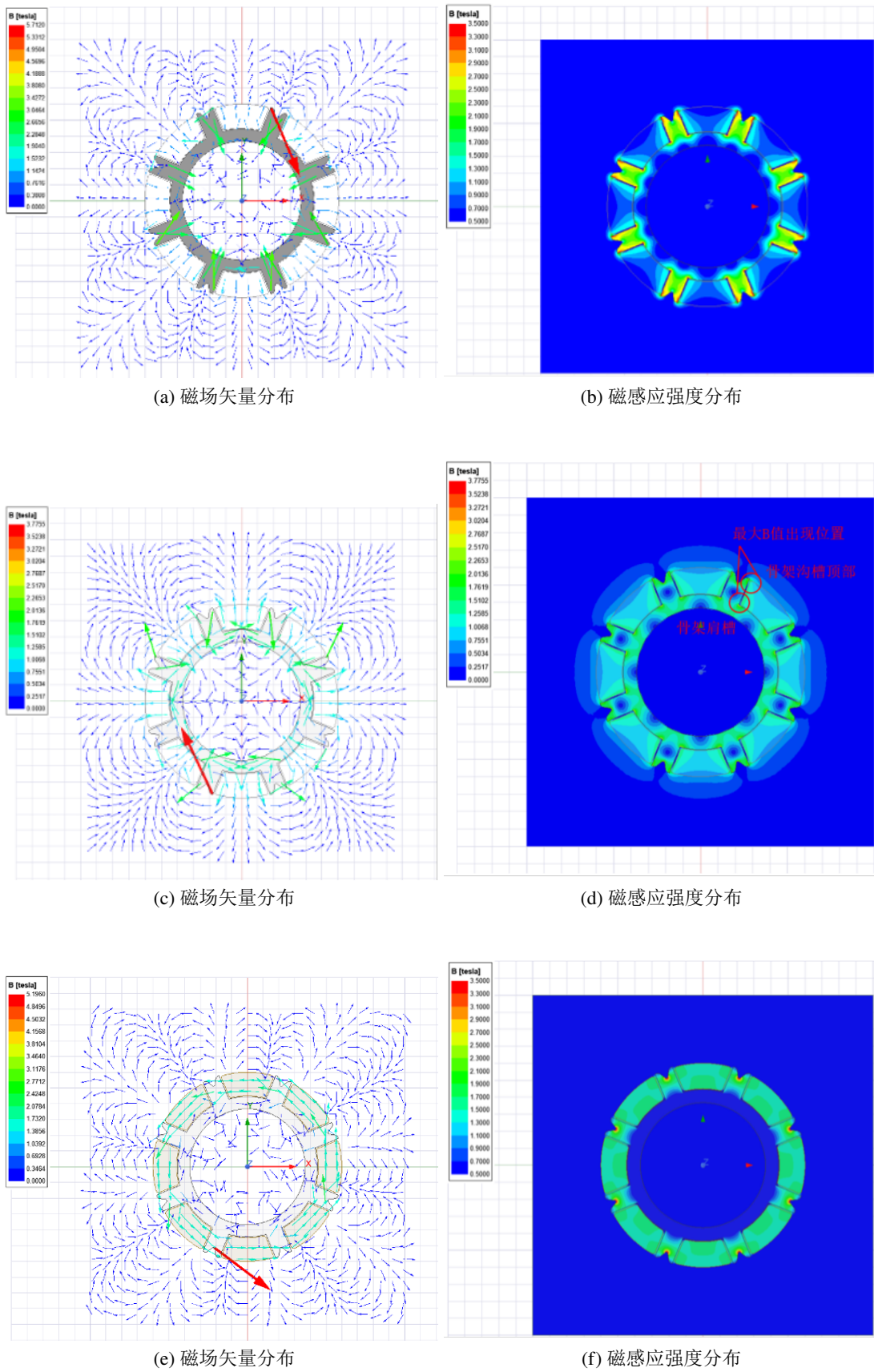
图 3.14: 磁铁采用不同磁化方式时下部强磁组件磁场计算结果
