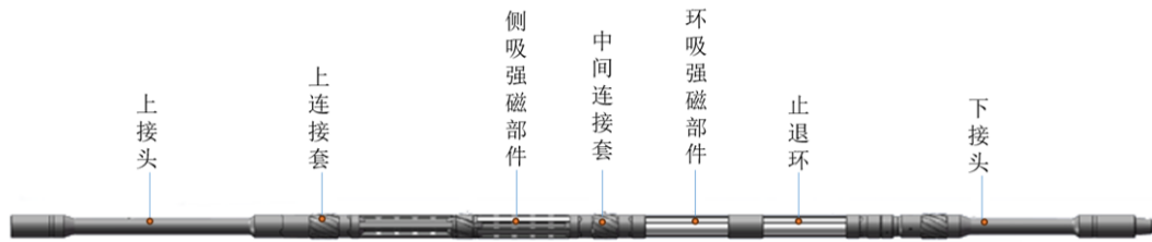
图 3.1: 大容量强磁吸附工具总体结构示意图
