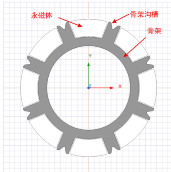
图 3.11: 强磁工具上部结构模型
