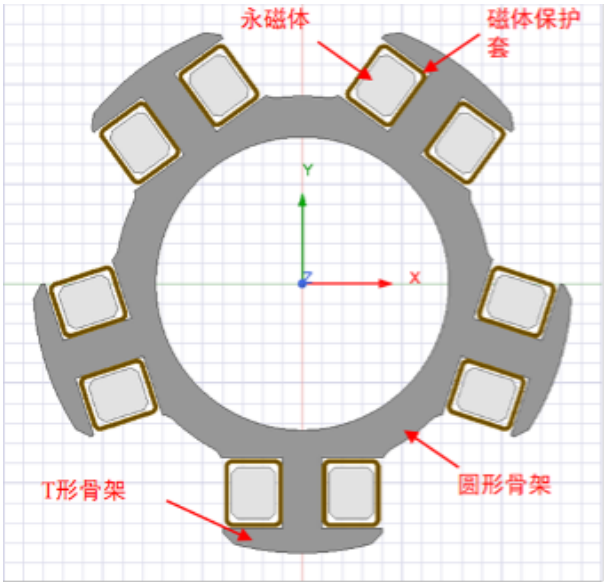
图 3.6: 强磁工具上部结构模型
