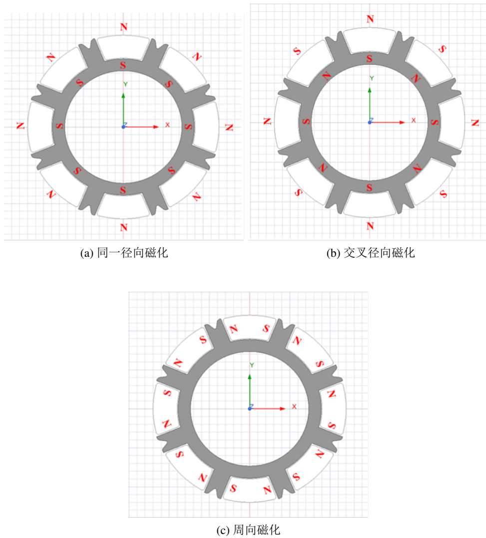
图 3.12: 下部强磁磁化方向示意图
