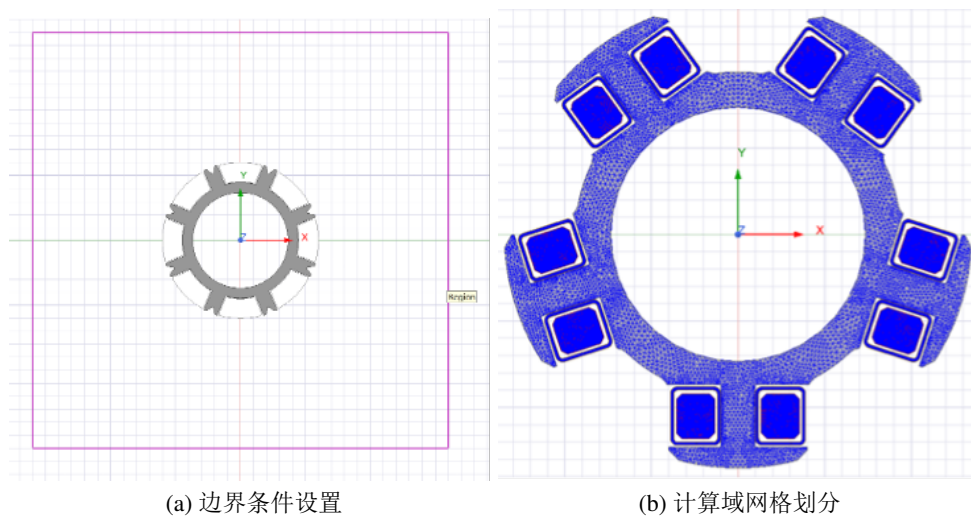
图 3.13: 下部强磁磁场分析设置
