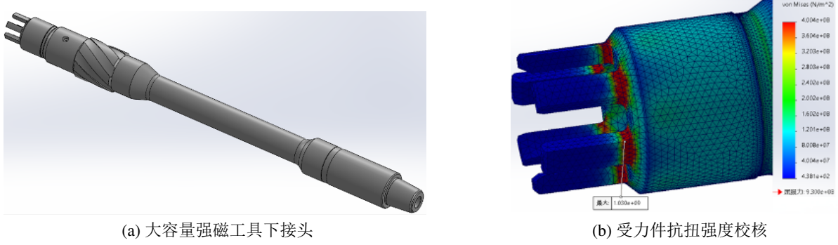
图 3.2: 受力件抗扭强度有限元分析结果
