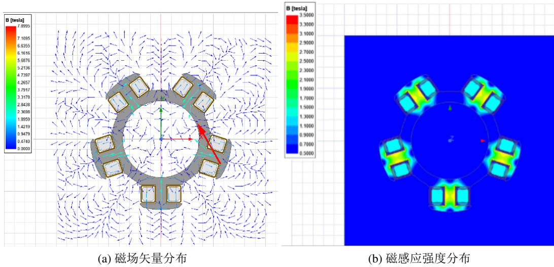
图 3.9: 磁铁径向磁化时上部强磁组件磁场计算结果
