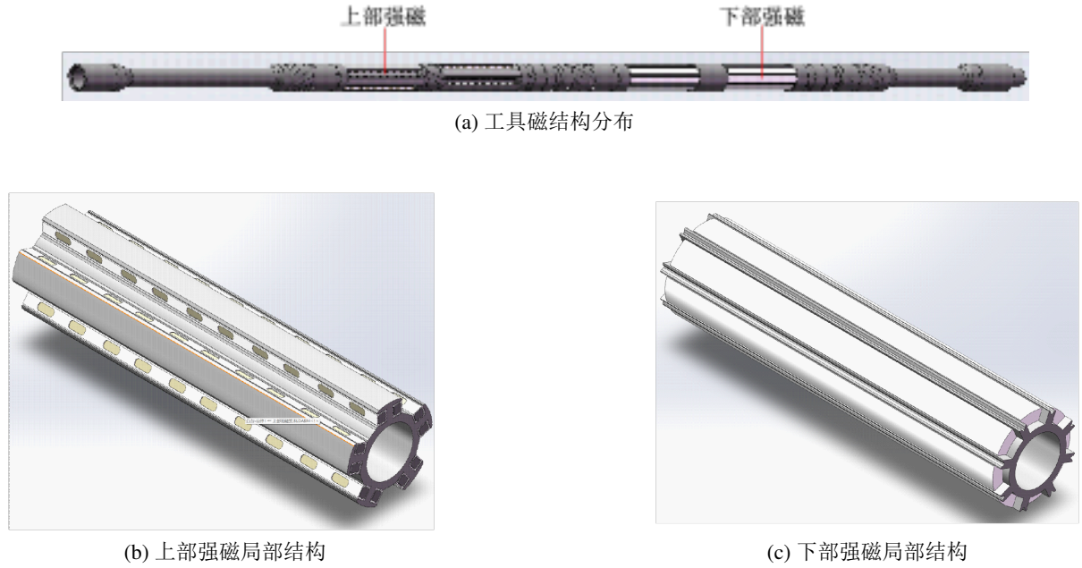
图 3.5: 大容量强磁工具含磁结构示意图
