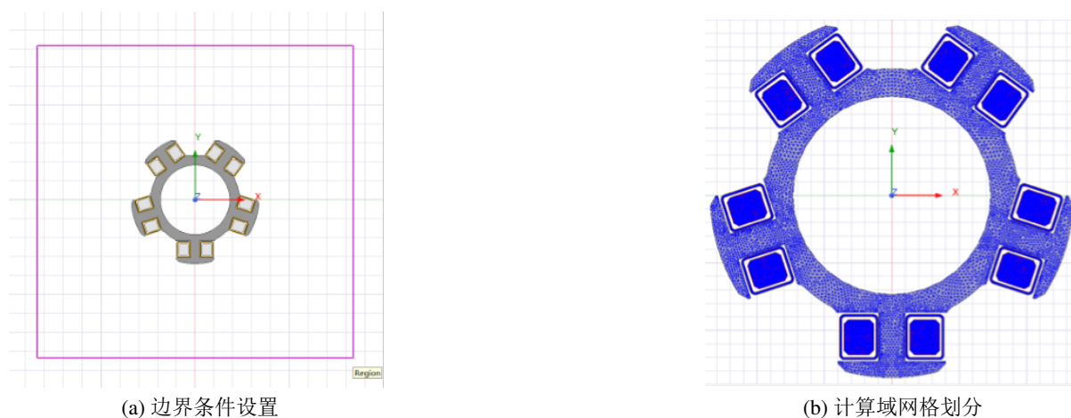
图 3.8: 上部强磁磁场分析设置
