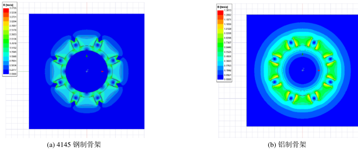
图 3.15: 骨架材料对磁场分布的影响
