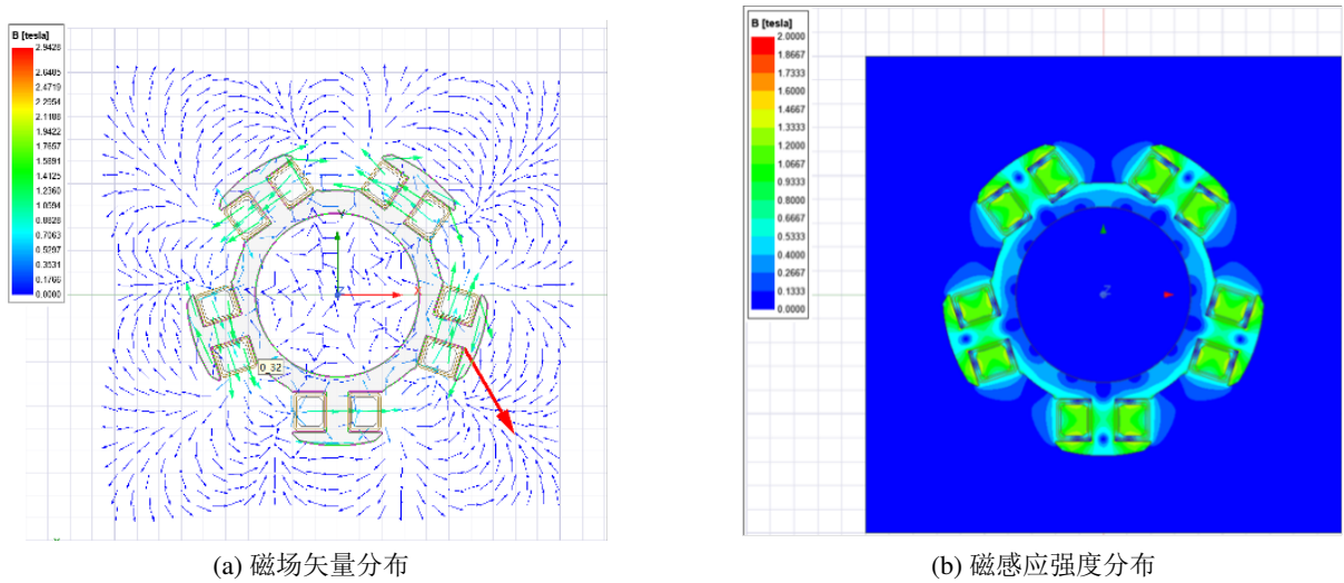
图 3.10: 磁铁周向磁化时上部强磁组件磁场计算结果
