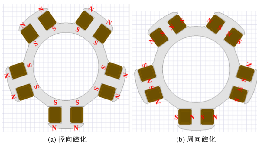
图 3.7: 上部强磁两种磁化方向示意图
