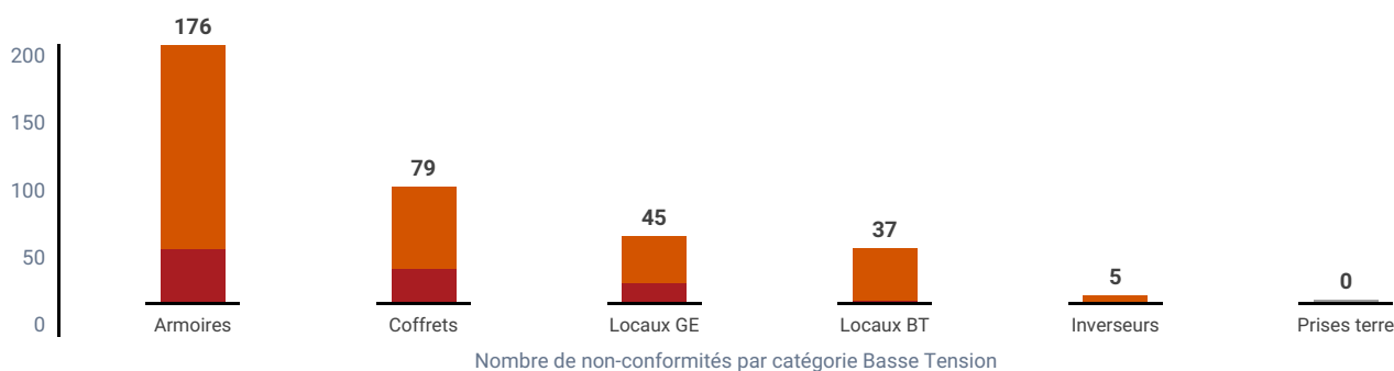
Non-conformités par catégorie - Basse Tension (BT)
