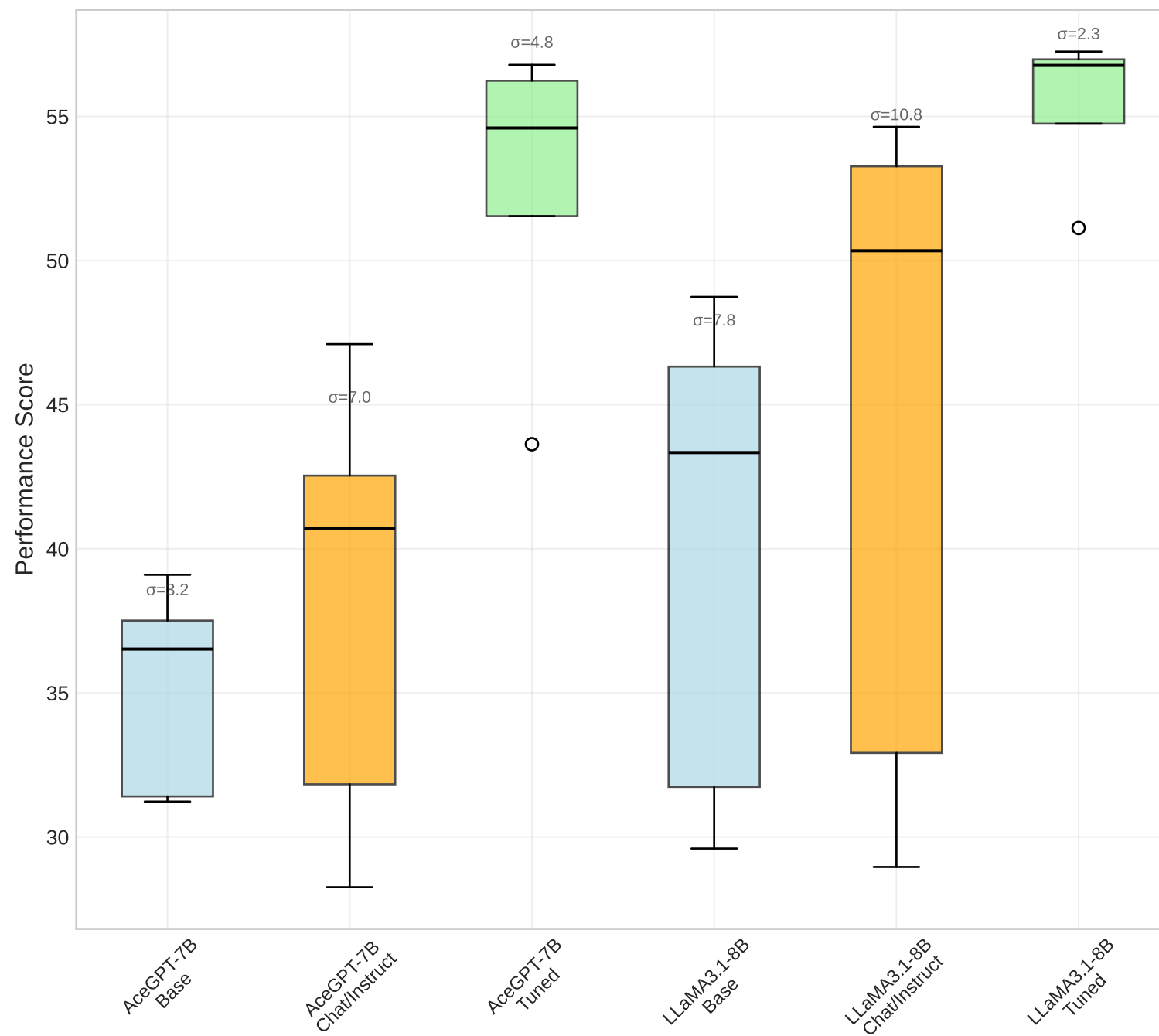
Intra-Dataset
