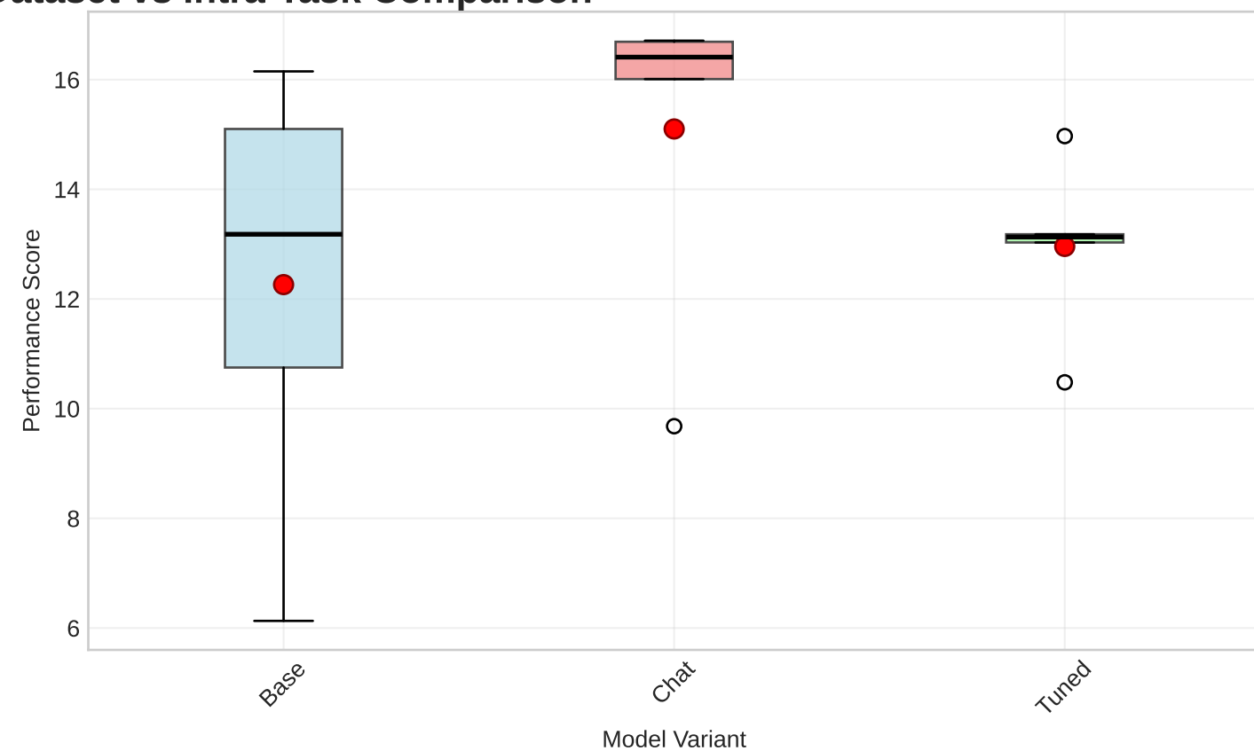
LLaMA3.1-8B - Intra-Task
