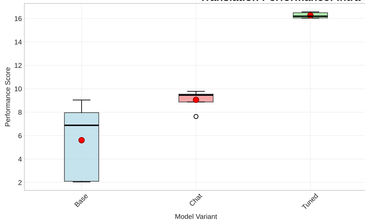
LLaMA3.1-8B - Intra-Dataset
