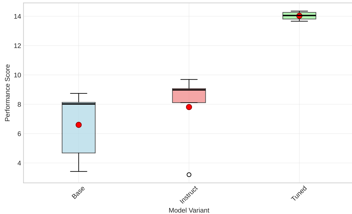
LLaMA3.1-8B - Intra-Dataset
