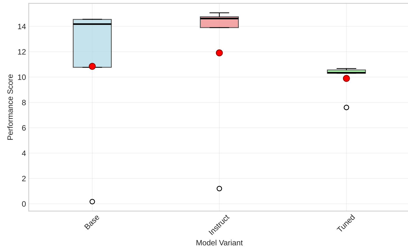
LLaMA3.1-8B - Intra-Task
