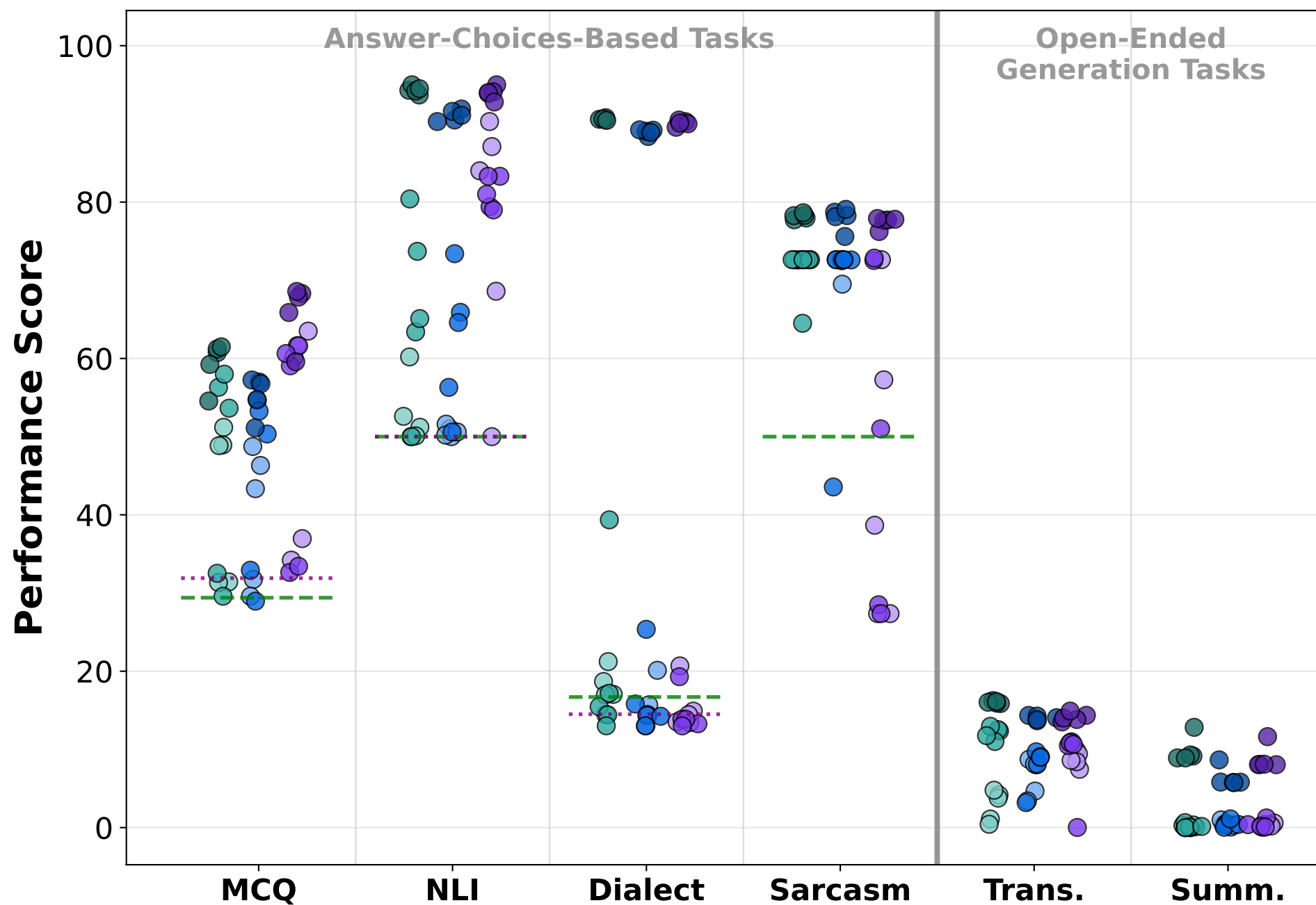
Intra-Dataset
