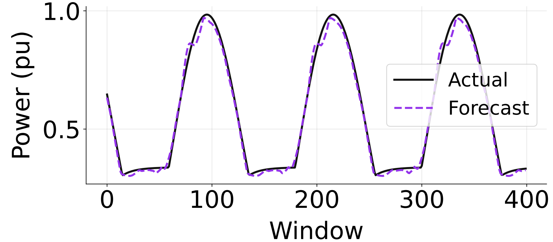
DC4 RMSE=0.023 pu
