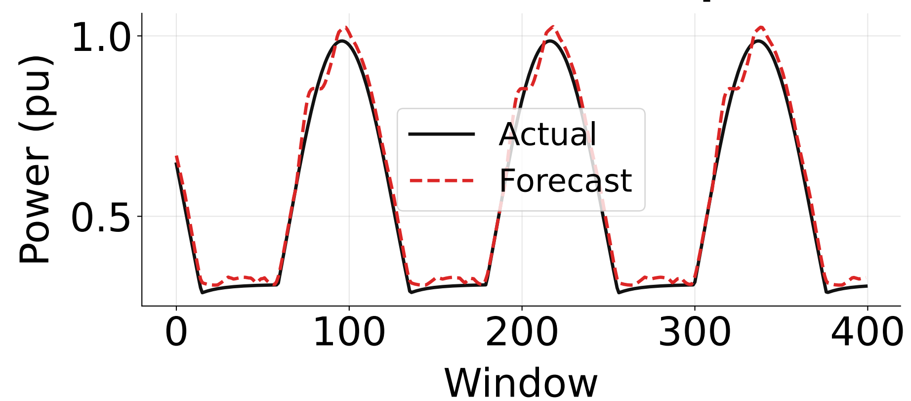
DC2 RMSE=0.029 pu
