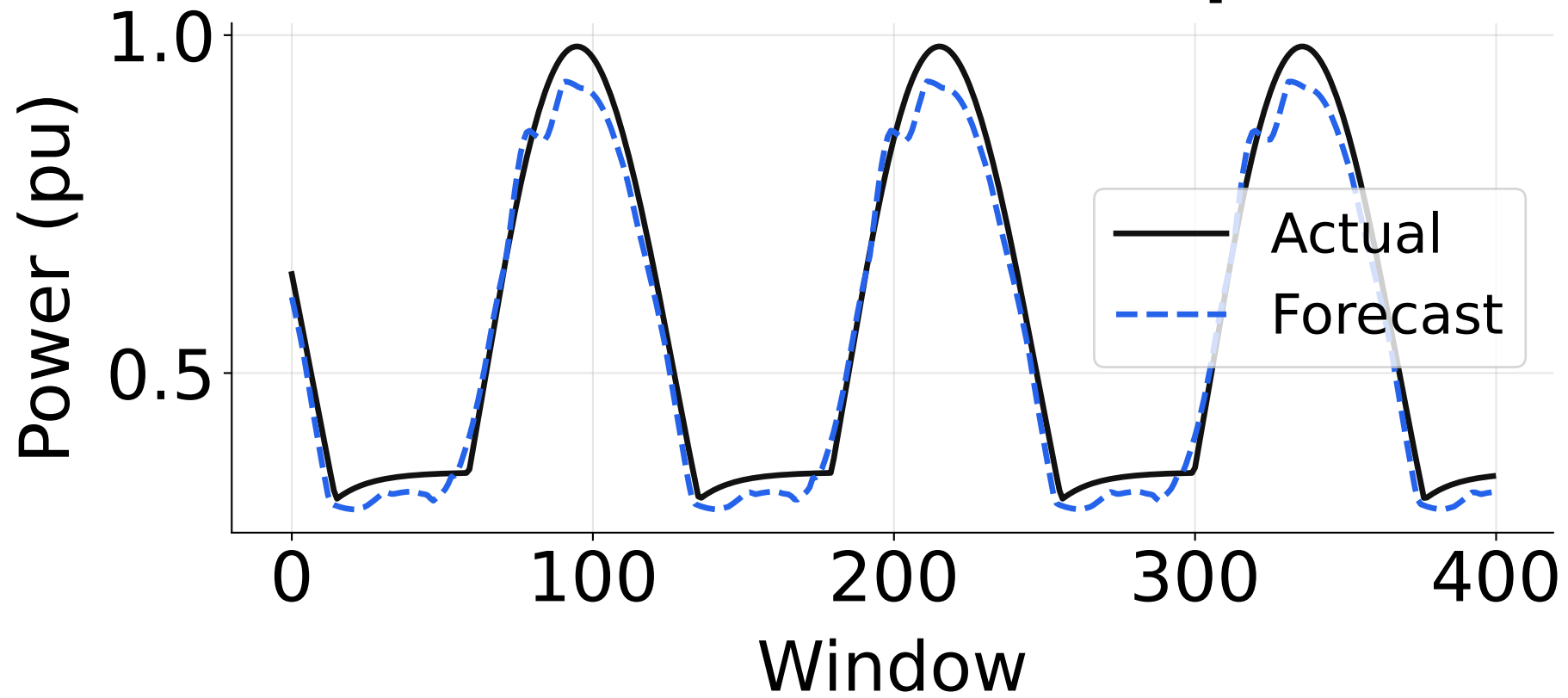
DC1 RMSE=0.038 pu
