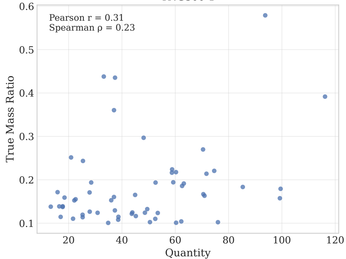
TNG300-1
