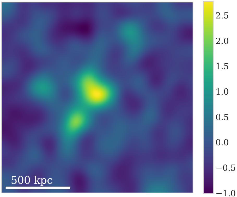
Aperture Mass S/N
