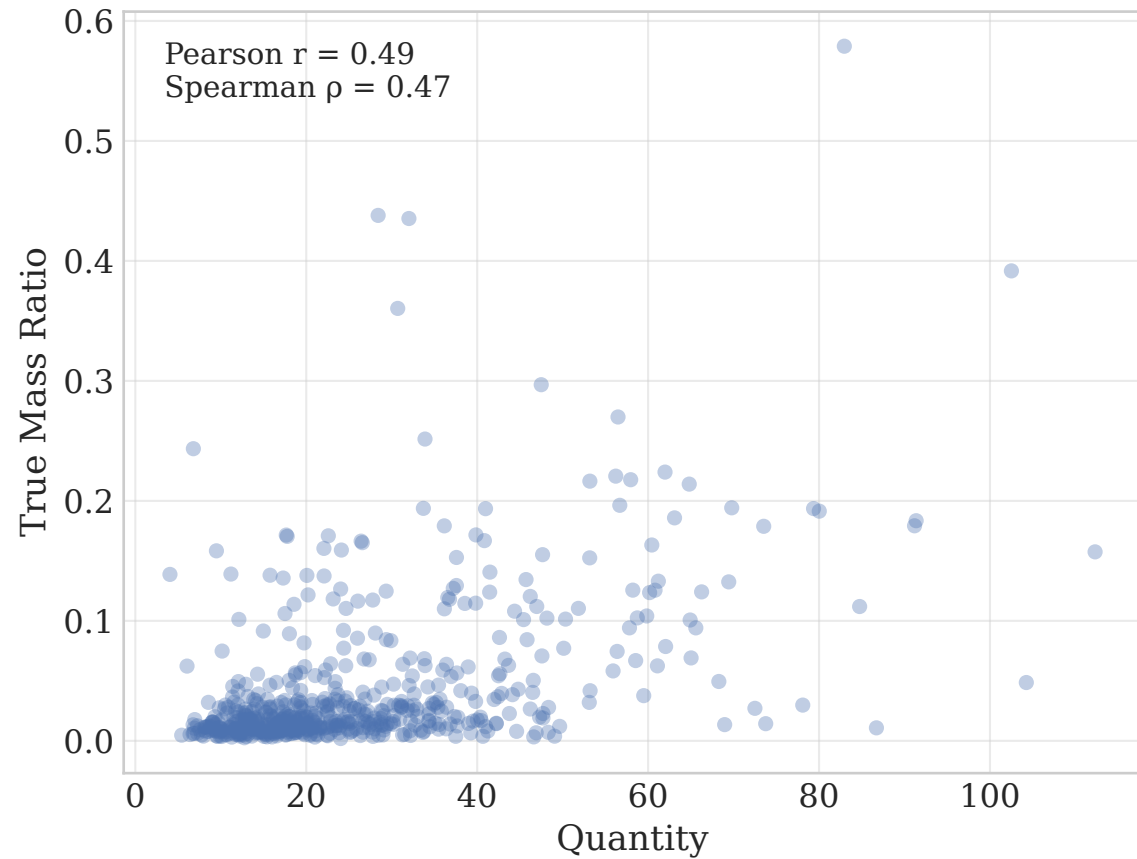
TNG300-1
