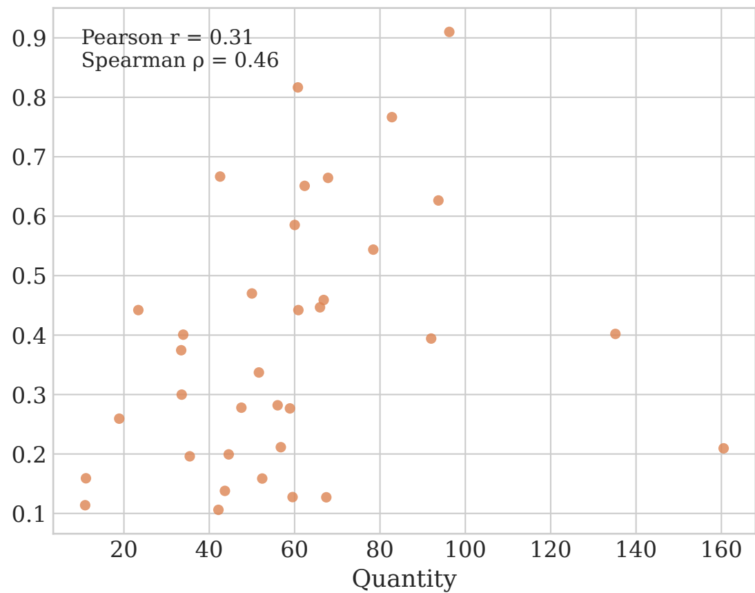
LoVoCCS
