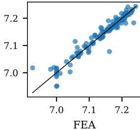
(d) min_fatigue_life_cycles (log10)
