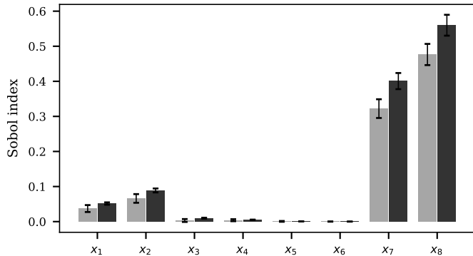
(b) Max. von Mises stress
