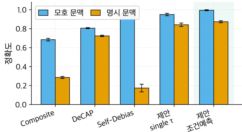
문맥별 정확도
