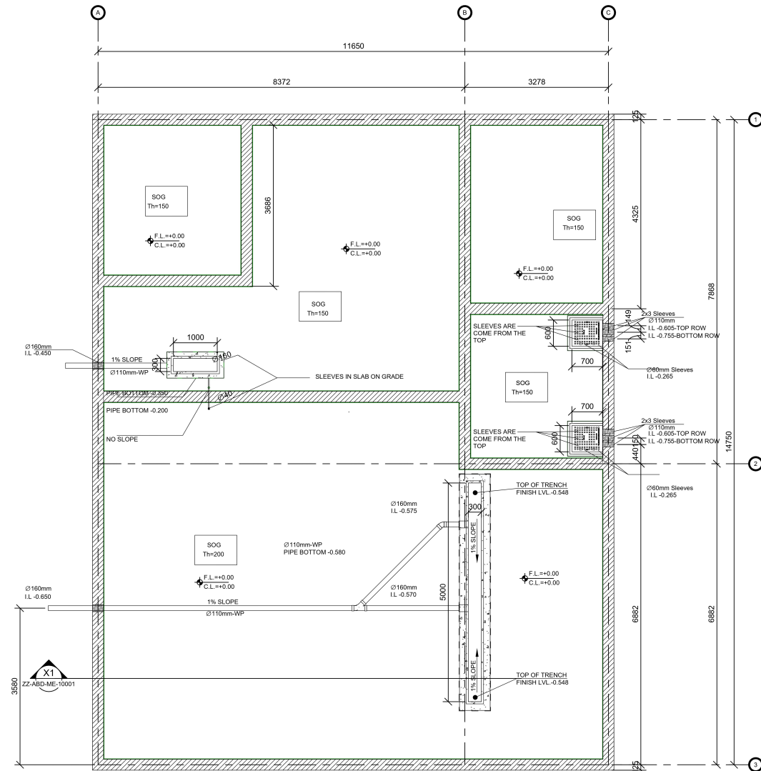
MEP SLEEVES LAYOUT 1 : 50
