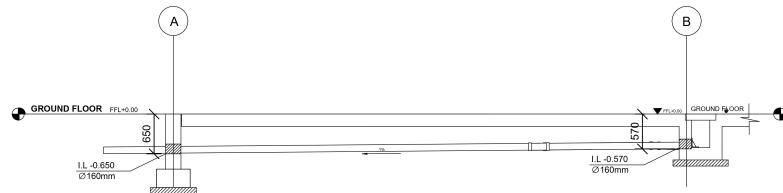
SECTION 1-1 1 : 50
