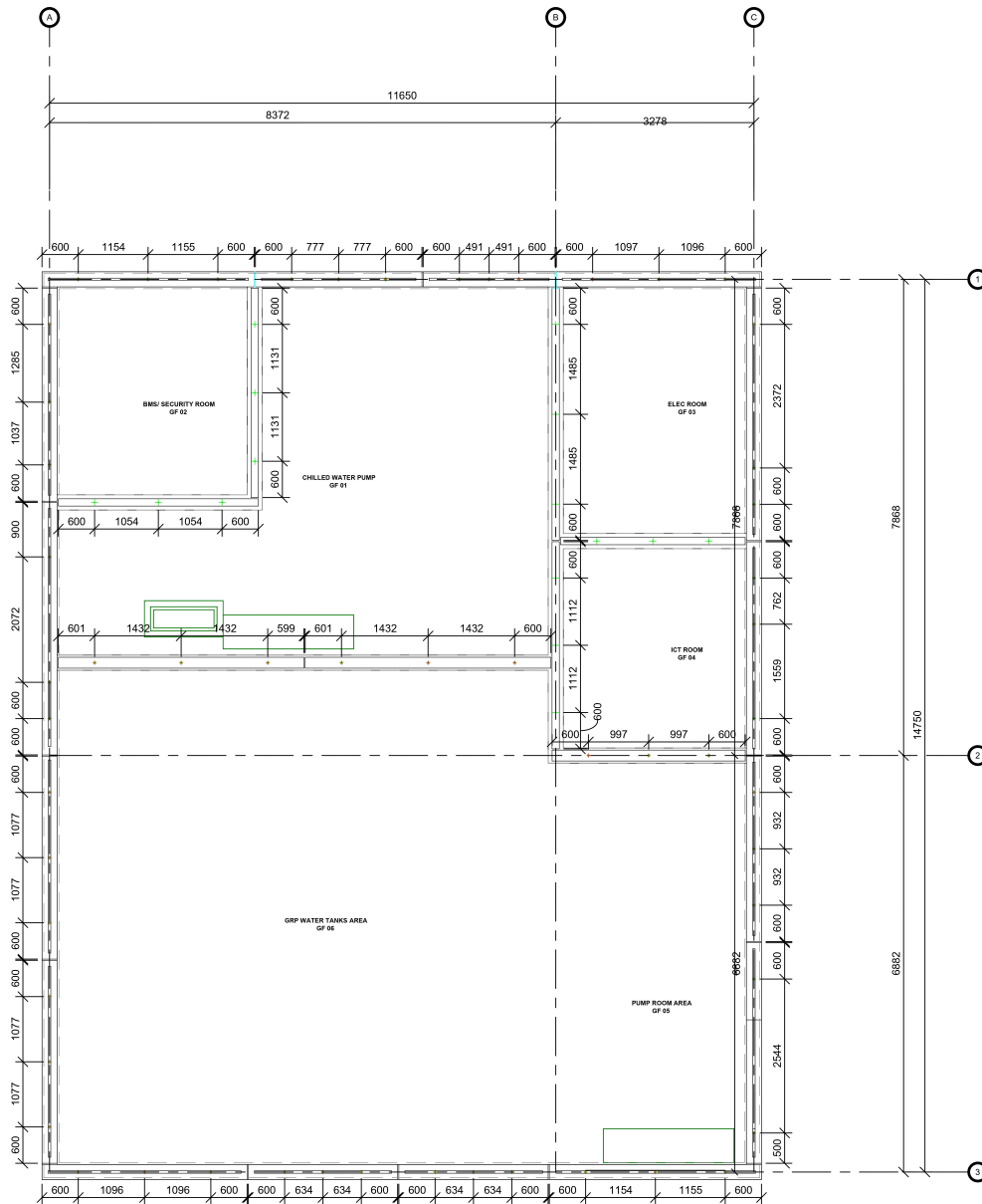
DOWEL LAYOUT 1 : 50
