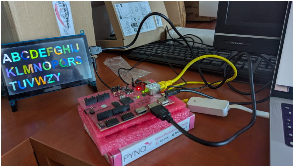
Figura 7: Implementarea fizica a sistemului: Placa PYNQ-Z1 conectata la ecranul LCD prin HDMI
