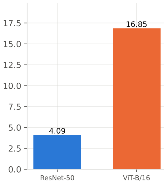
compute (GMACs)
