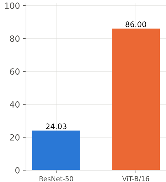
parameters (M)
