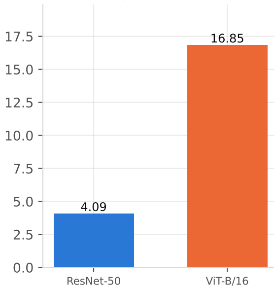
compute (GMACs)
