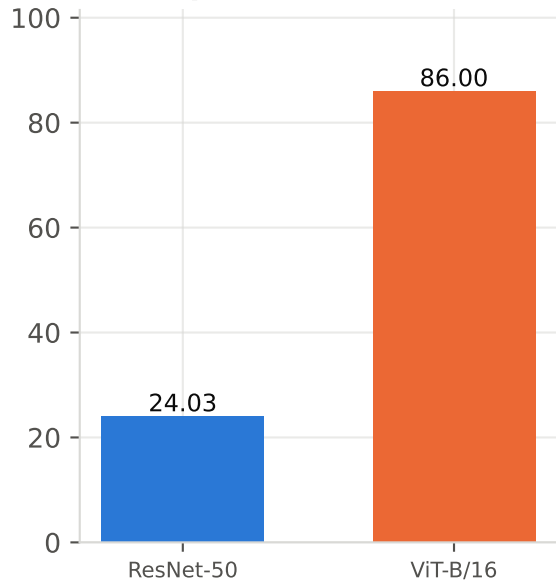
parameters (M)
