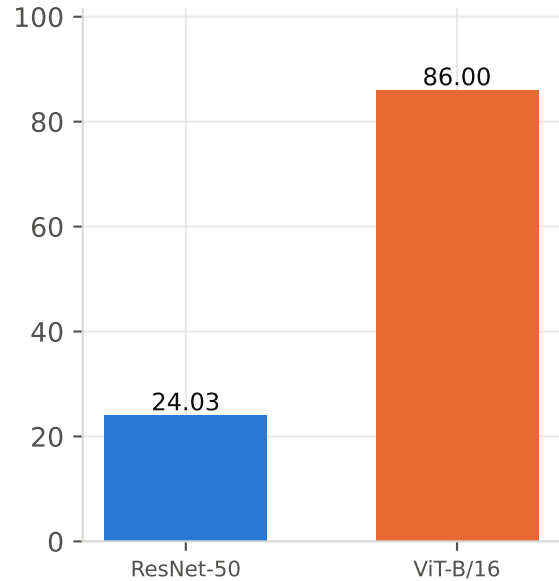
parameters (M)
