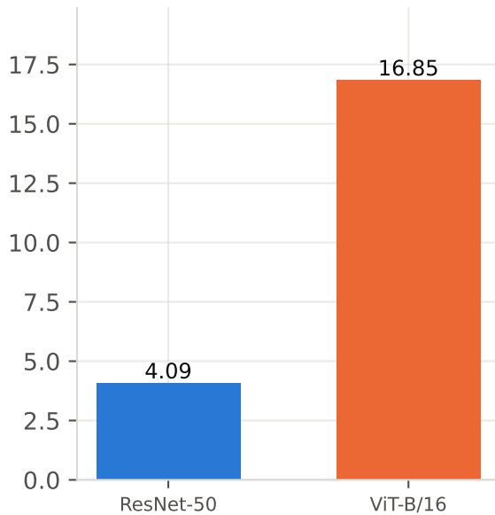
compute (GMACs)
