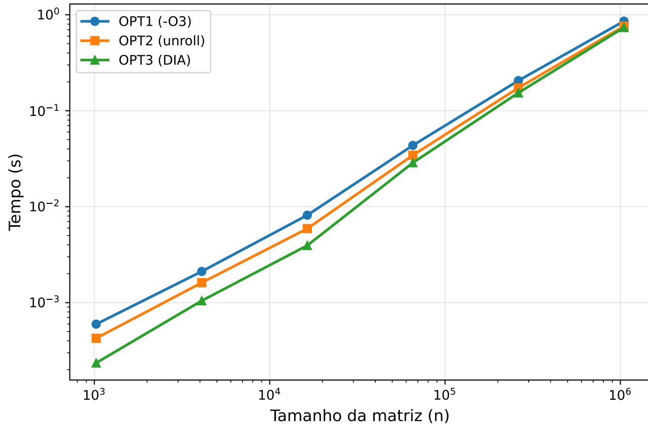
Tempo de Execução - Bandas=27
