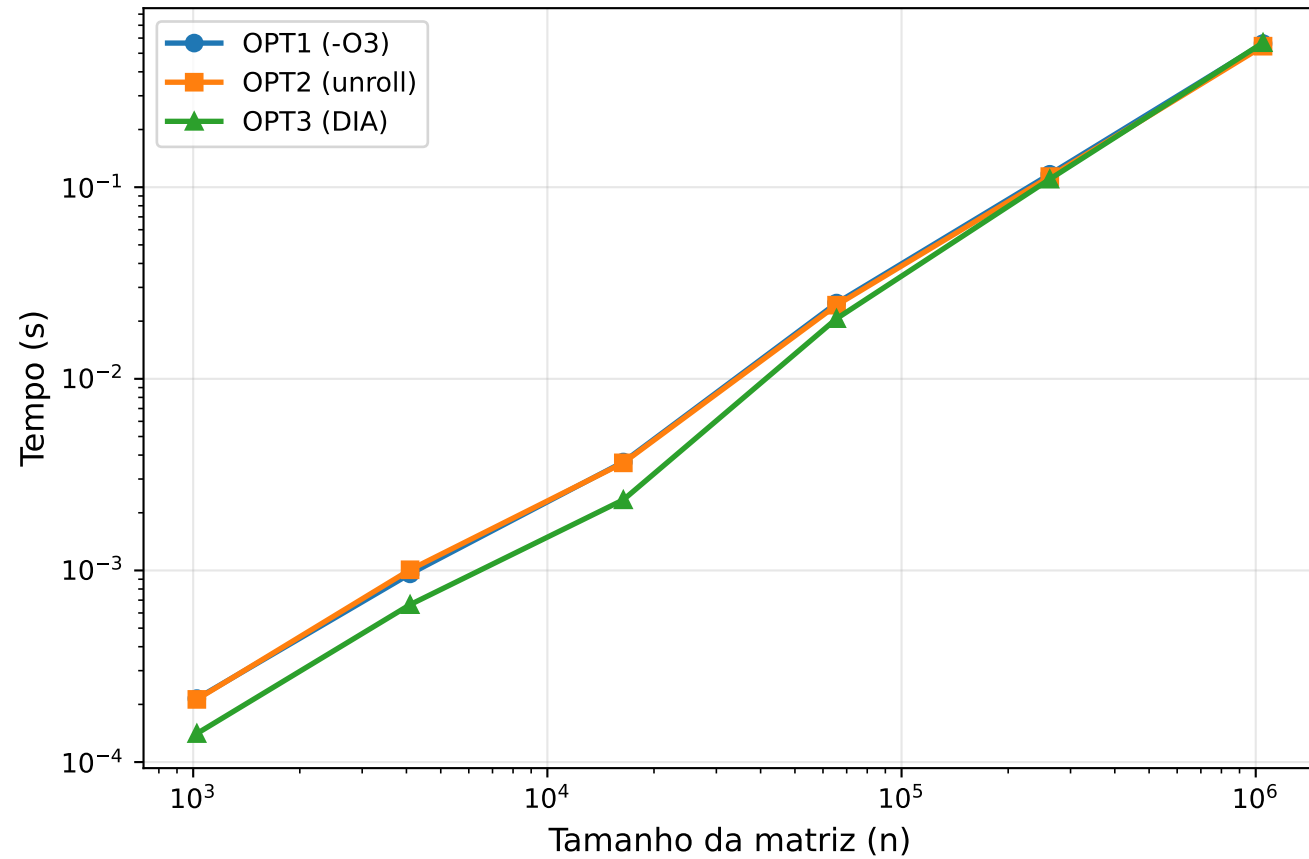
Tempo de Execução - Bandas=7
