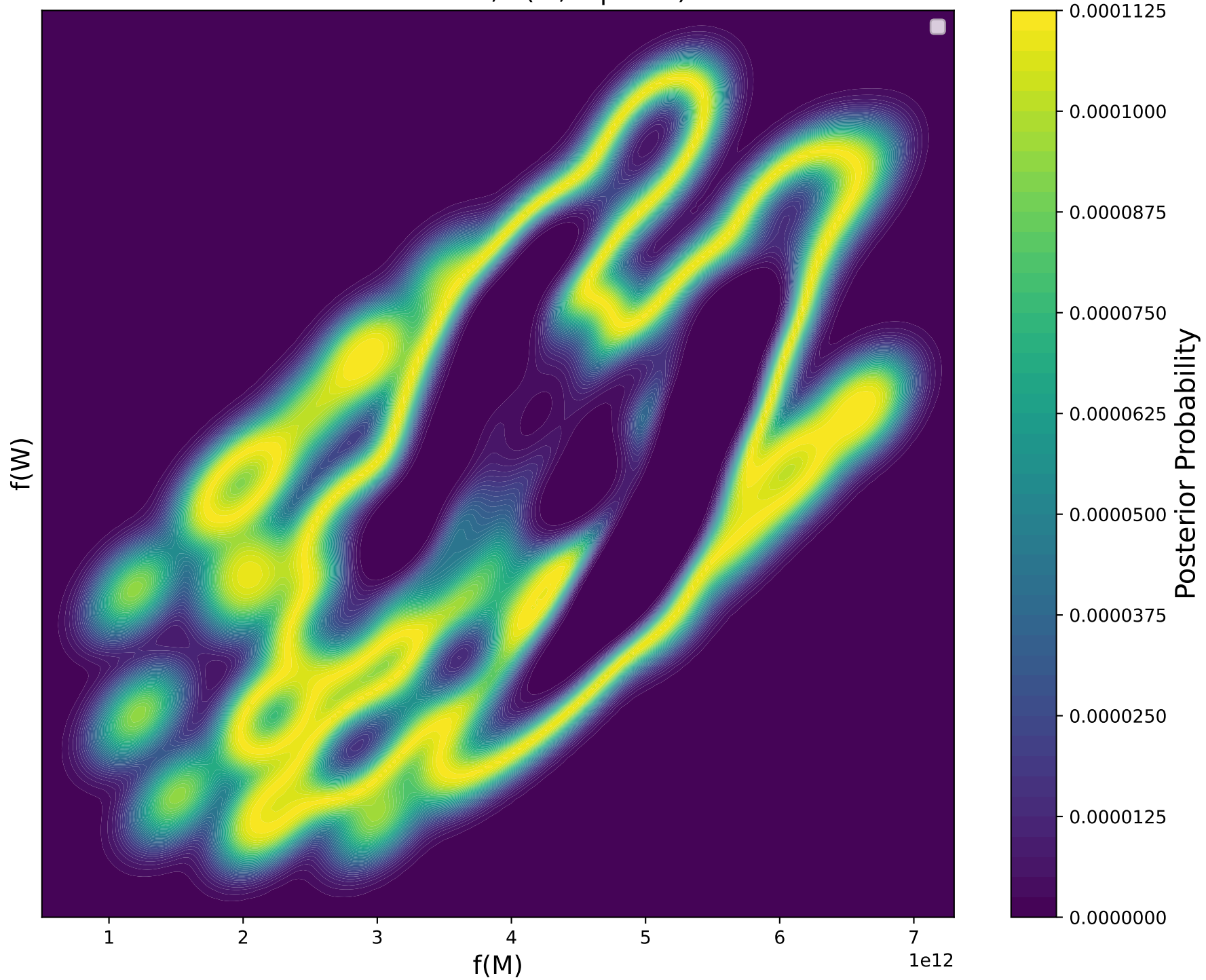
Posterior PDF, \pi(M, W|X = 1)
