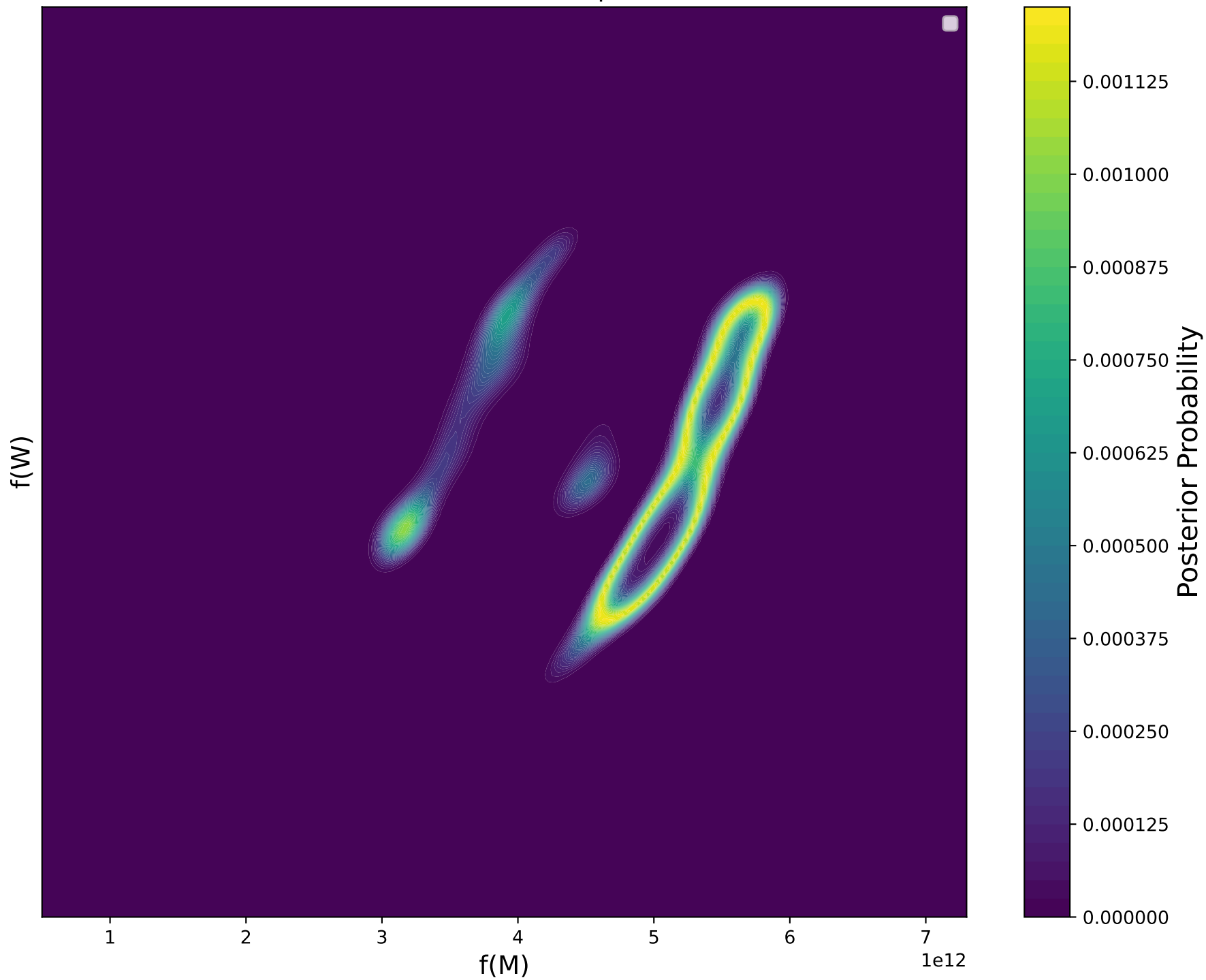
Posterior PDF, \pi(M, W|X = 17)
