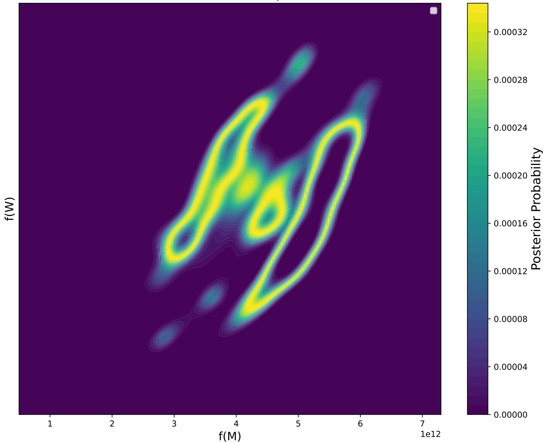
Posterior PDF, \pi(M, W|X = 8)
