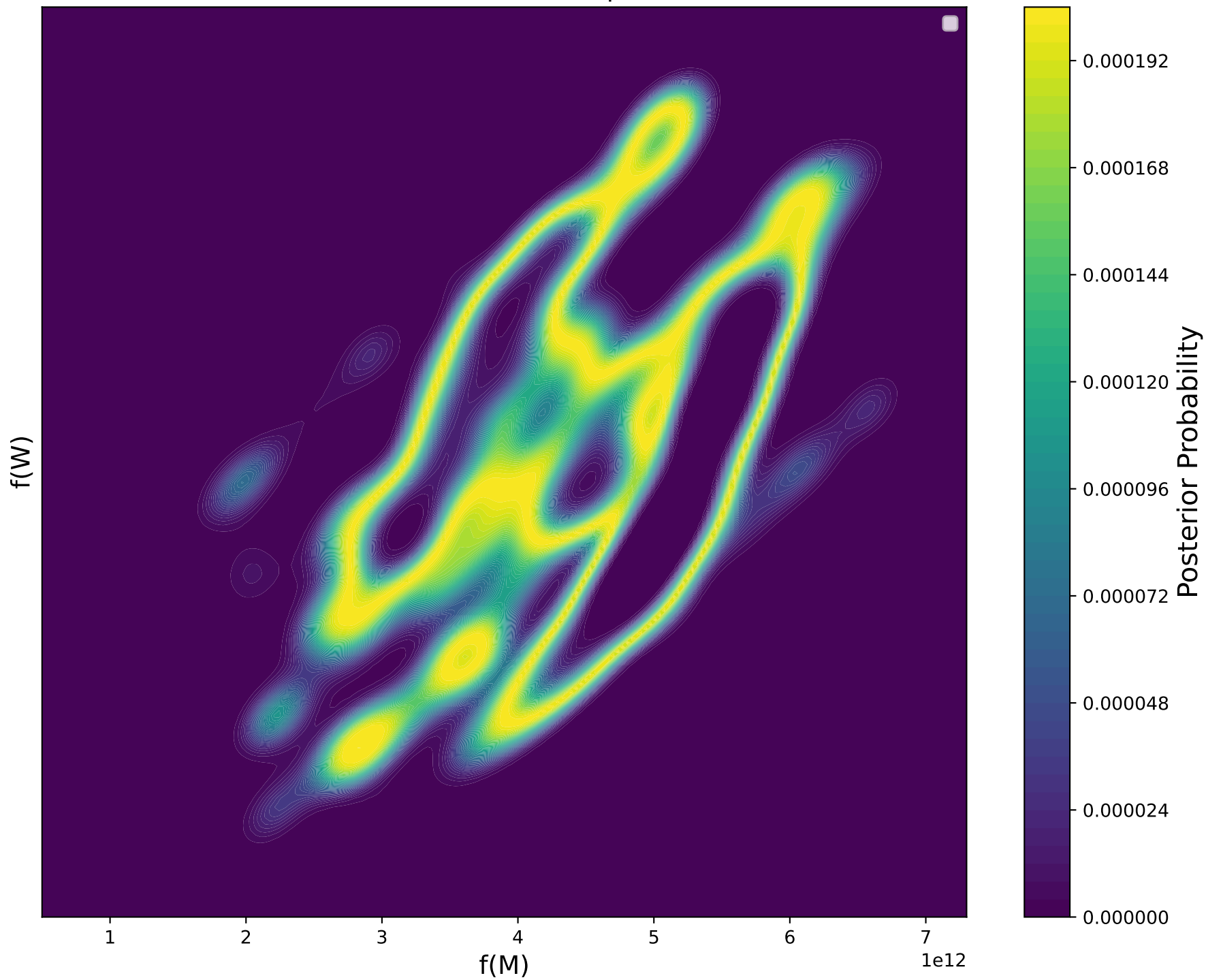
Posterior PDF, \pi(M, W|X = 4)
