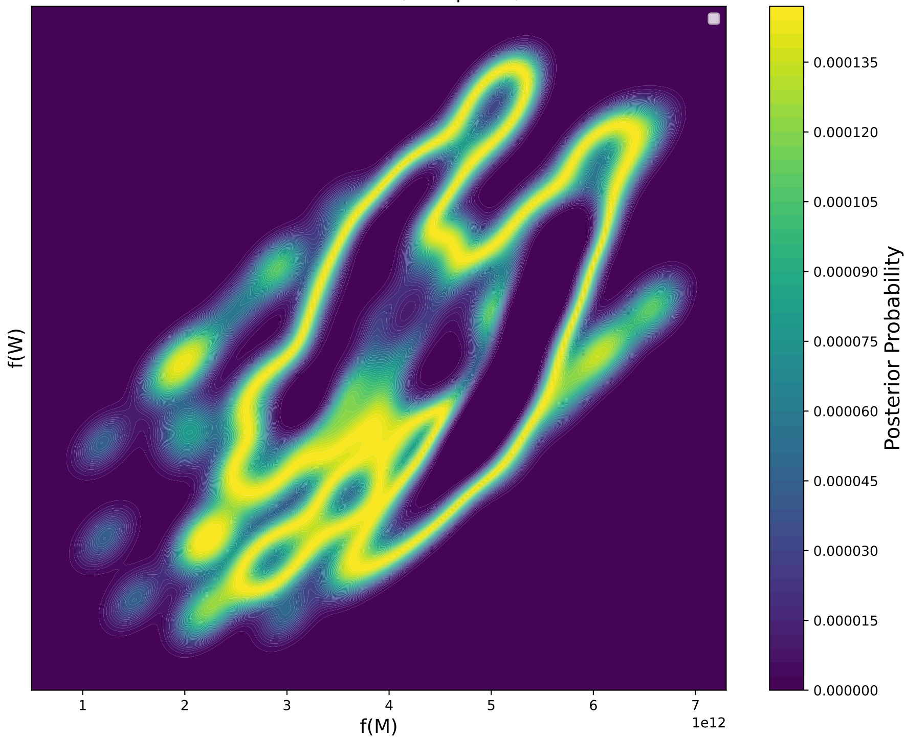
Posterior PDF, \pi(M, W|X = 2)
