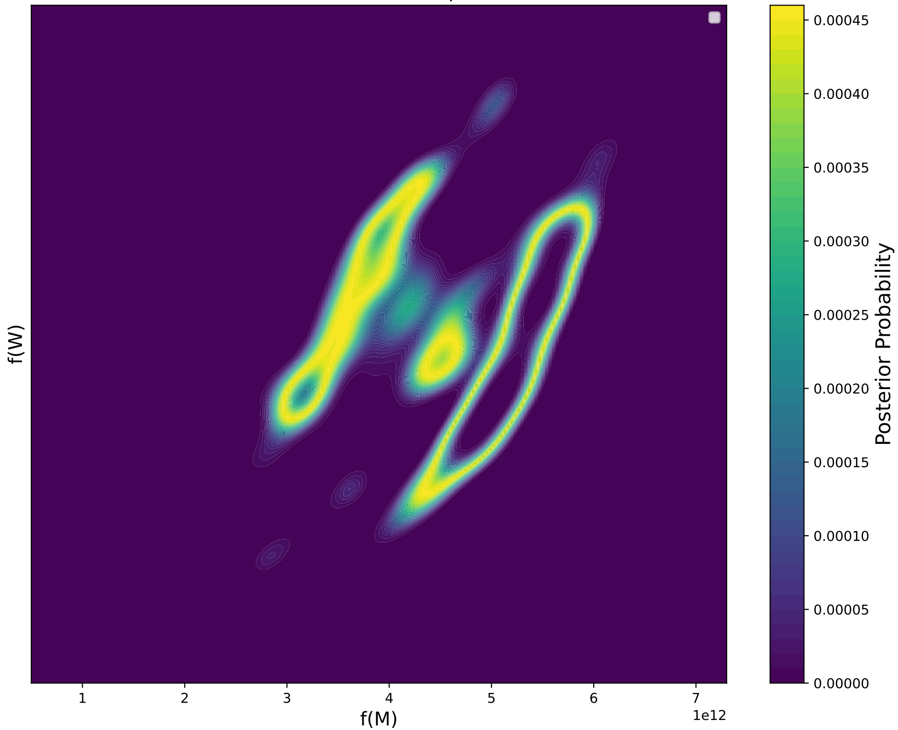
Posterior PDF, \pi(M, W|X = 10)
