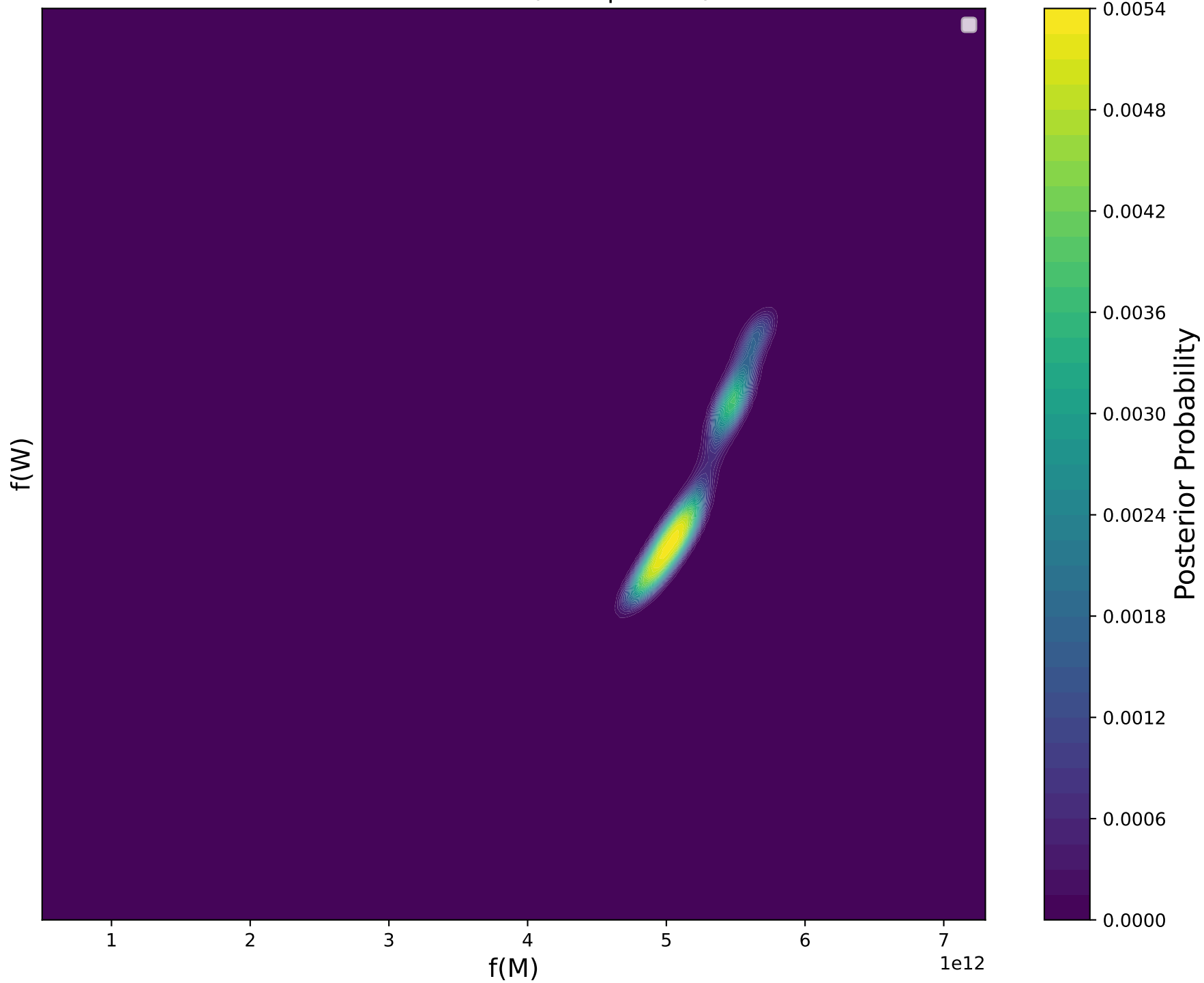
Posterior PDF, \pi(M, W|X = 31)
