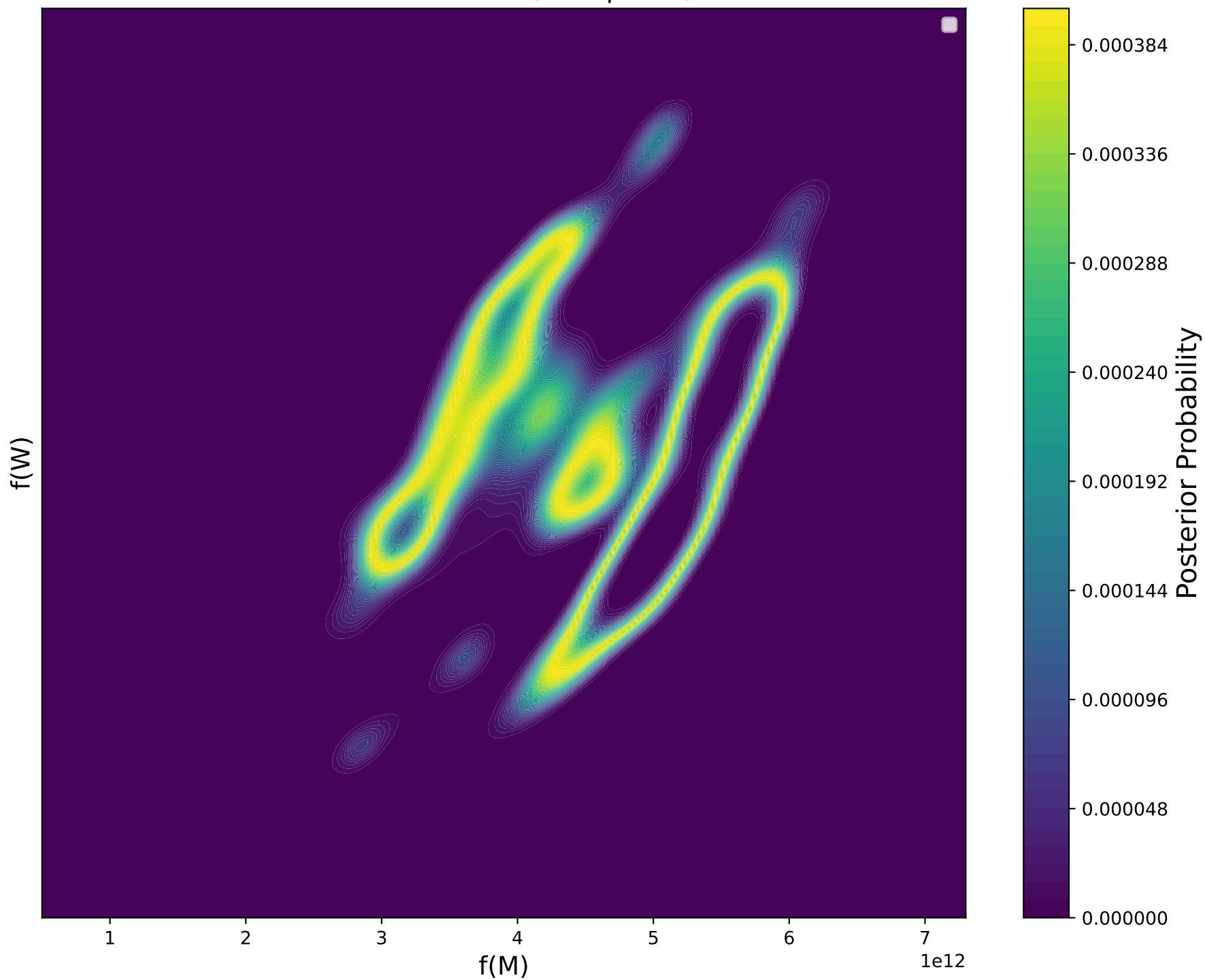
Posterior PDF, \pi(M, W|X = 9)
