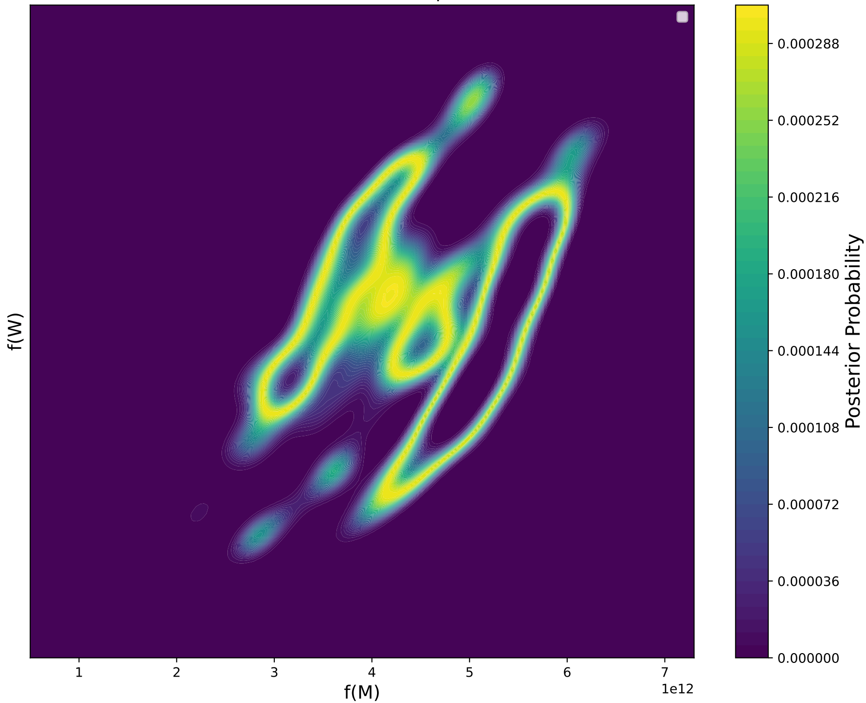
Posterior PDF, \pi(M, W|X = 7)
