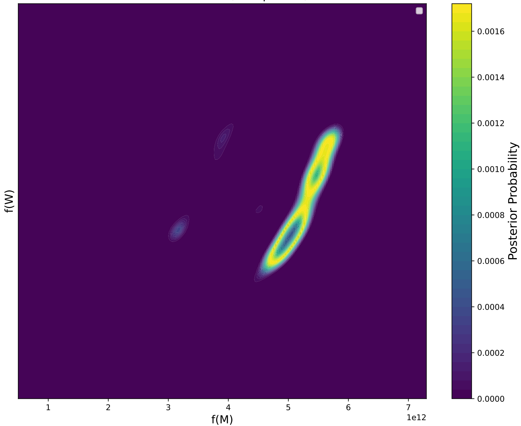
Posterior PDF, \pi(M, W|X = 22)
