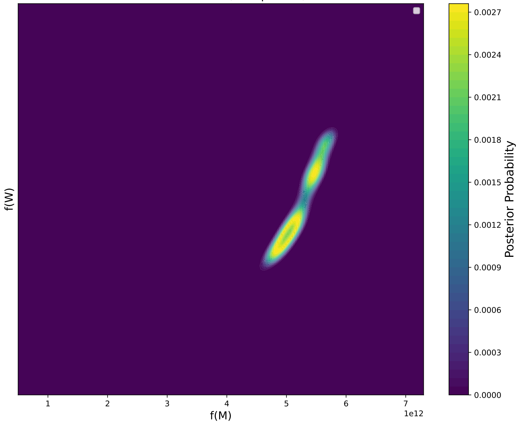
Posterior PDF, \pi(M, W|X = 27)
