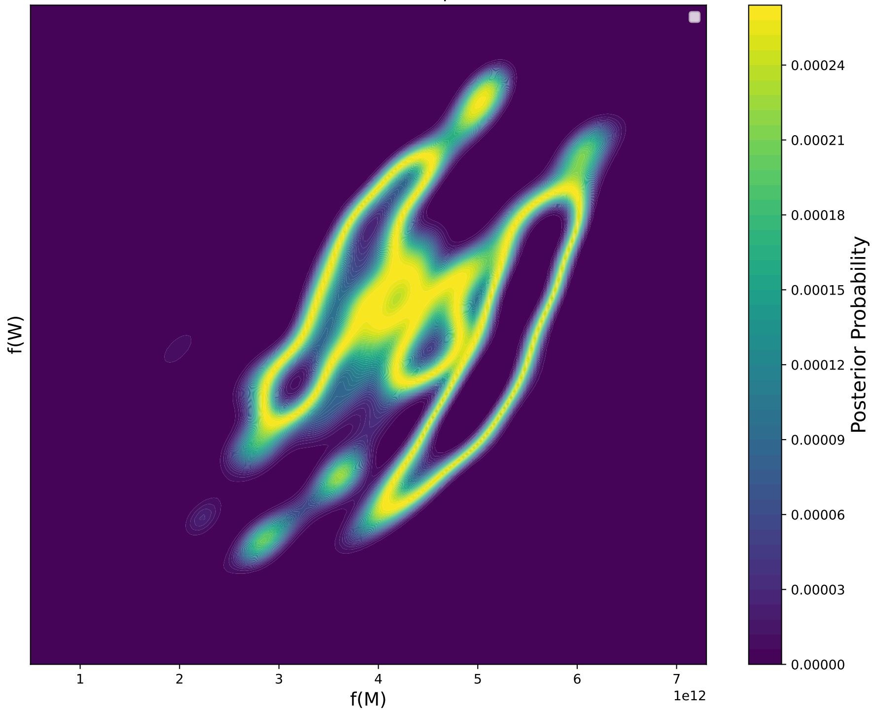
Posterior PDF, \pi(M, W|X = 6)
