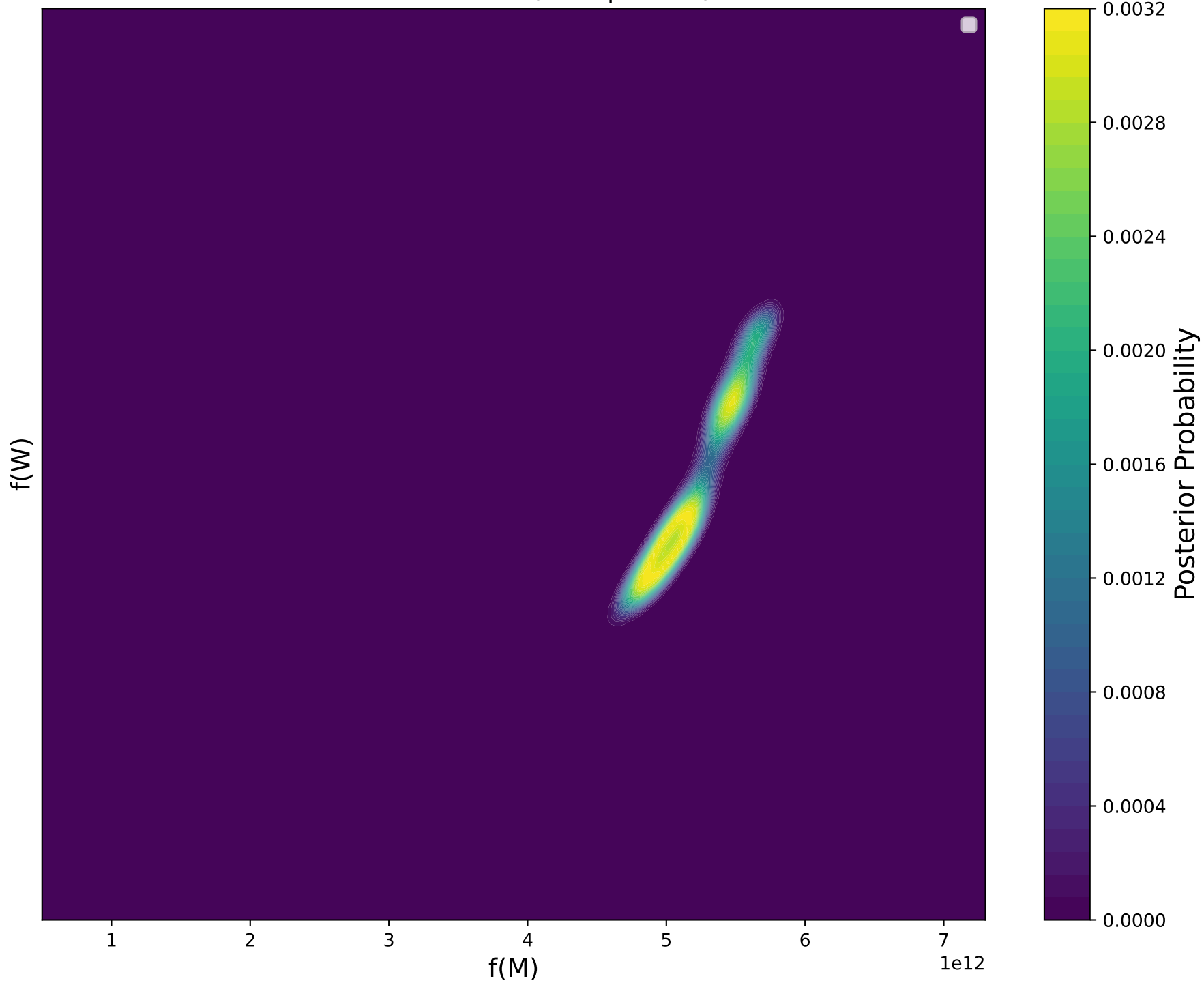
Posterior PDF, \pi(M, W|X = 28)
