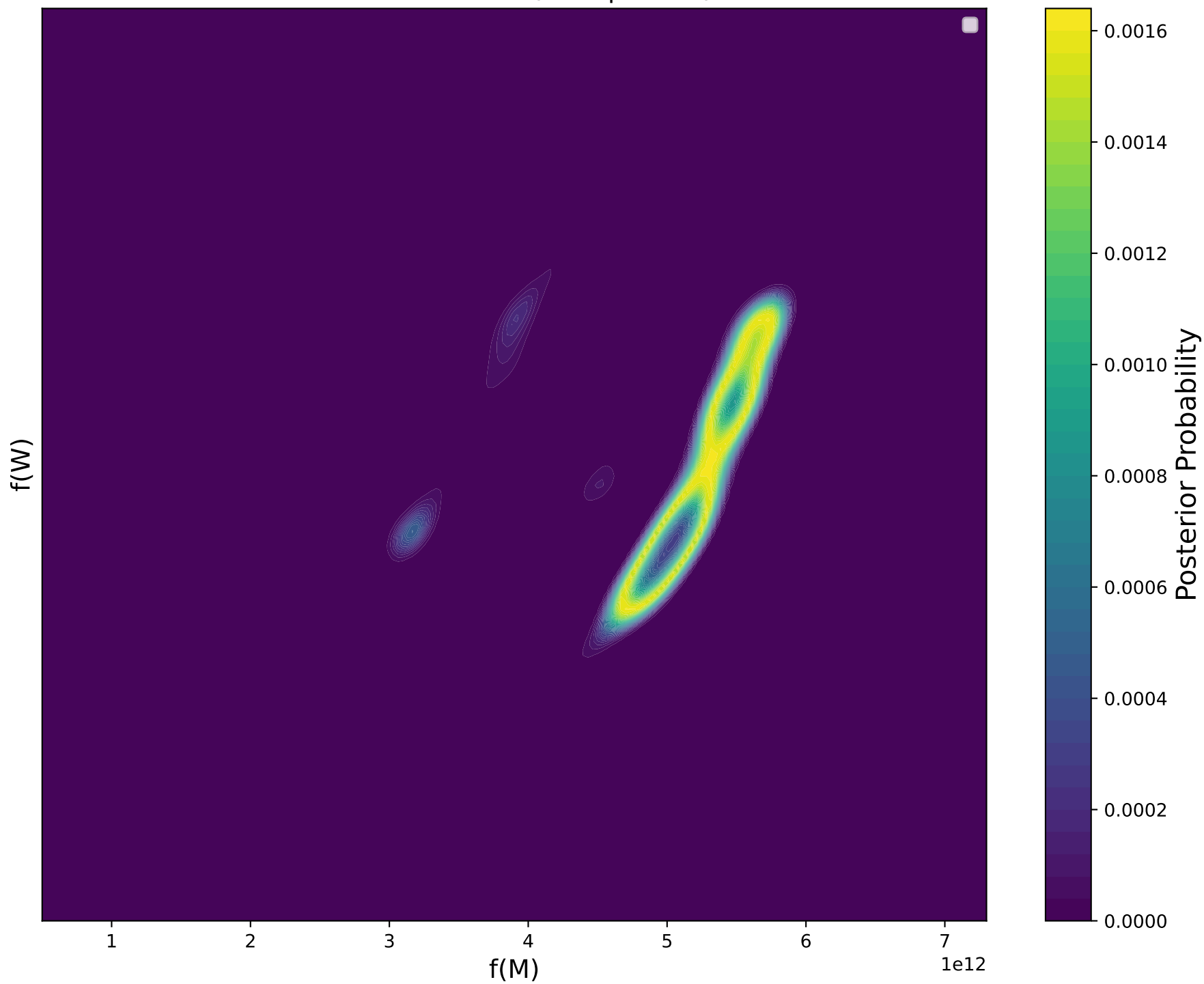
Posterior PDF, \pi(M, W|X = 21)
