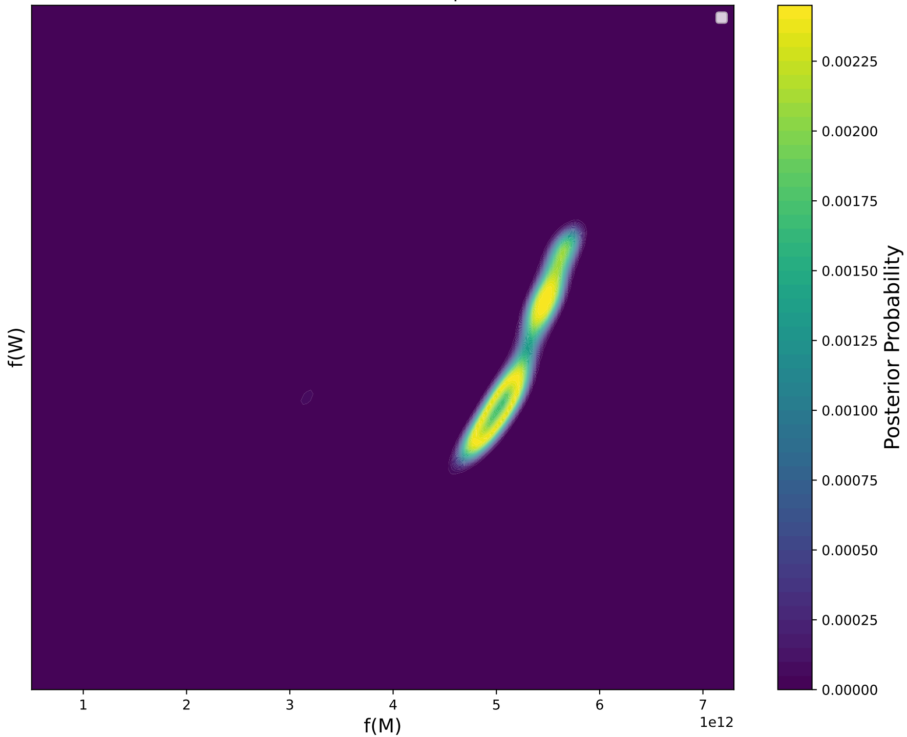
Posterior PDF, \pi(M, W|X = 26)
