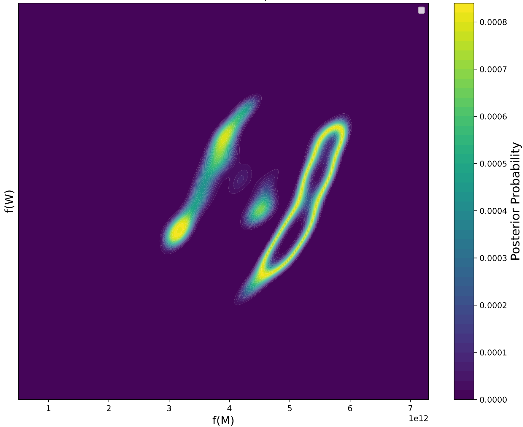
Posterior PDF, \pi(M, W|X = 14)
