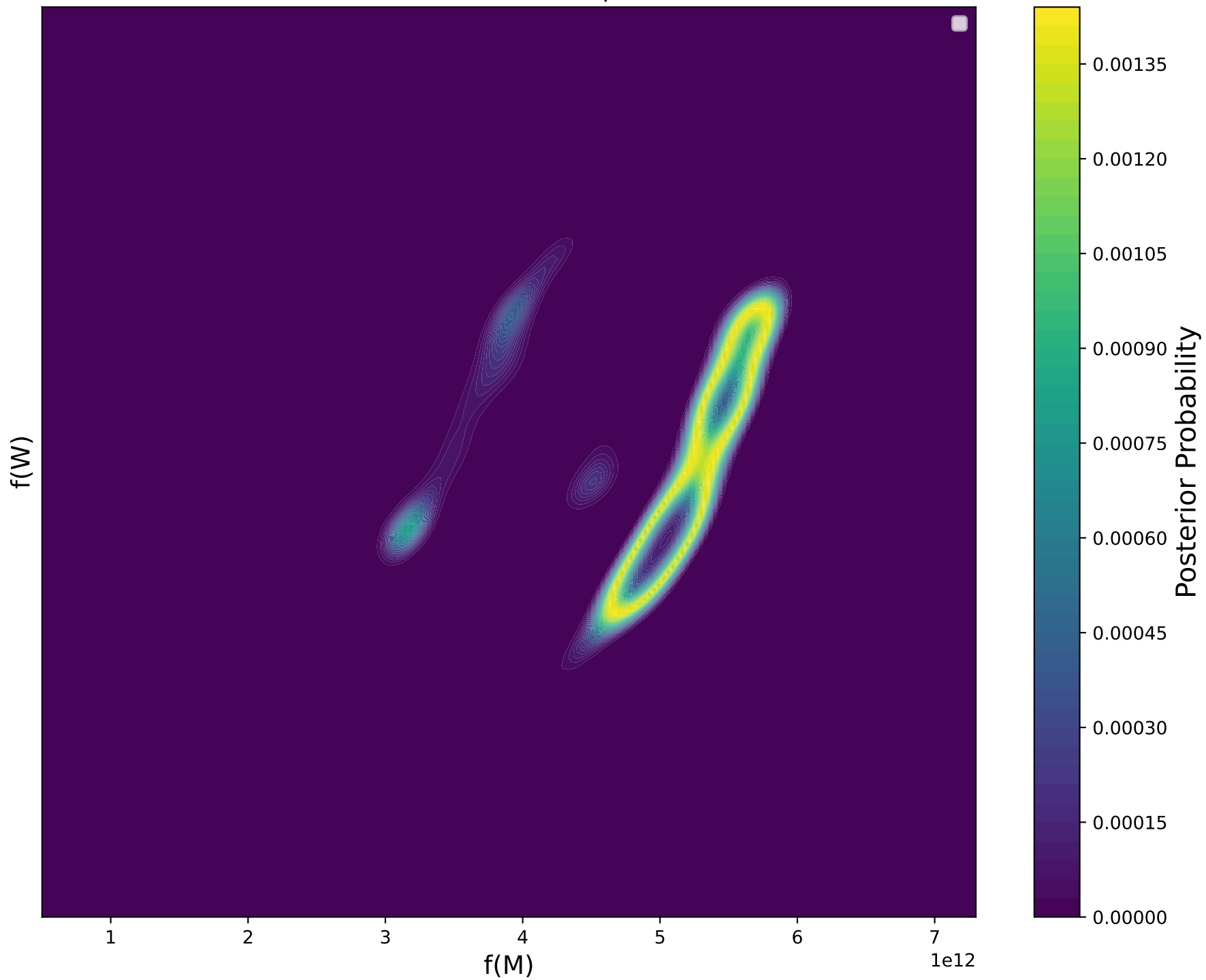
Posterior PDF, \pi(M, W|X = 19)
