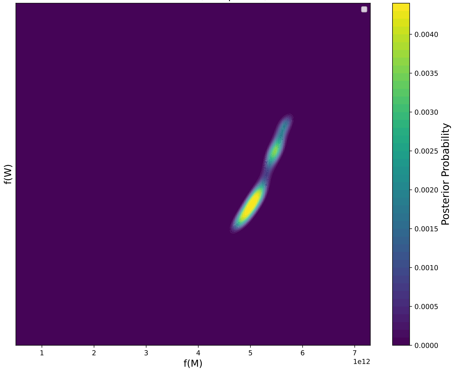
Posterior PDF, \pi(M, W|X = 30)
