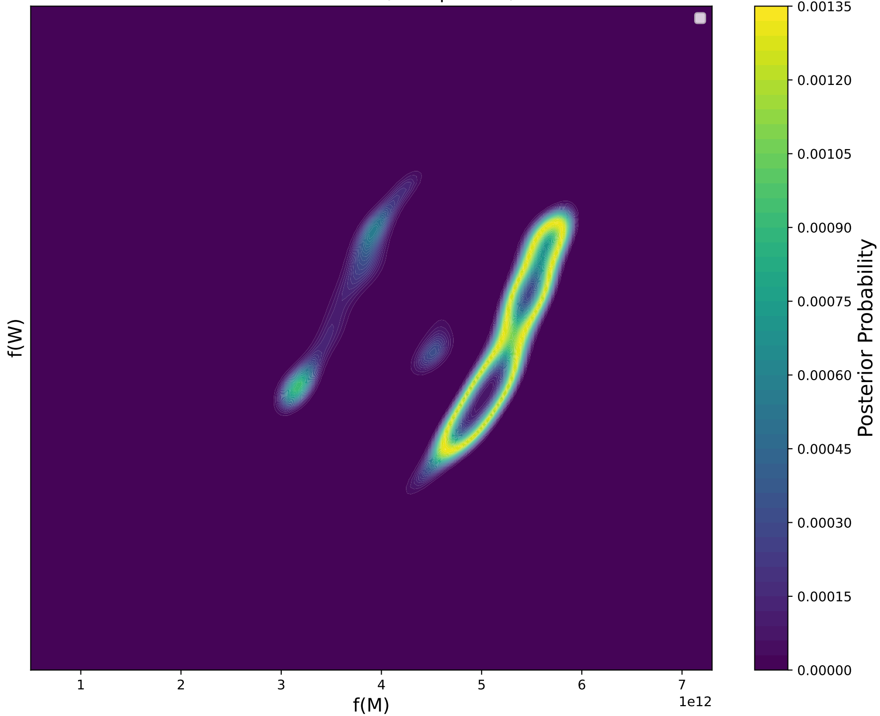
Posterior PDF, \pi(M, W|X = 18)
