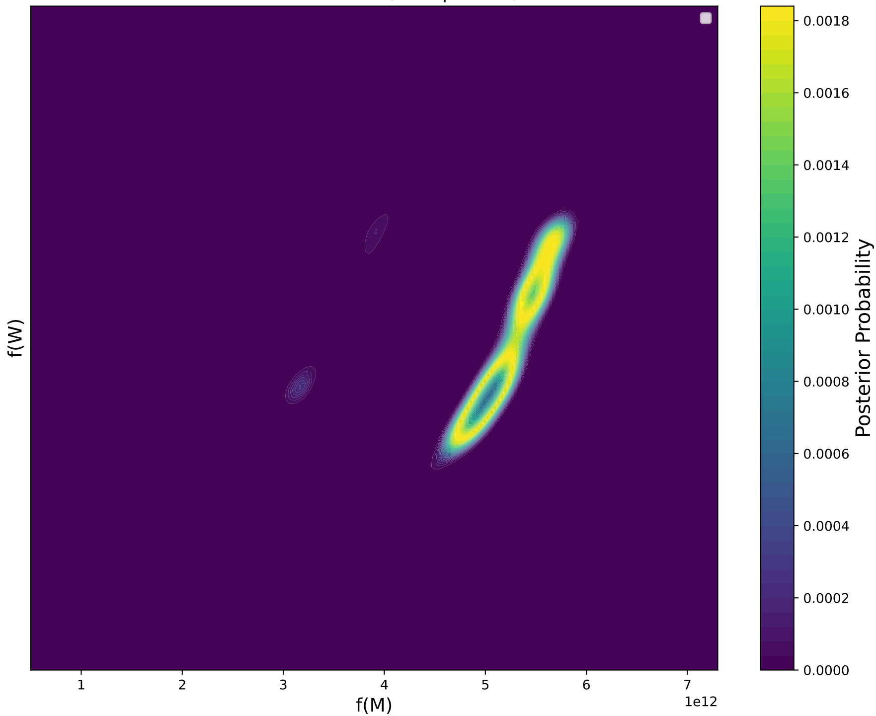
Posterior PDF, \pi(M, W|X = 23)
