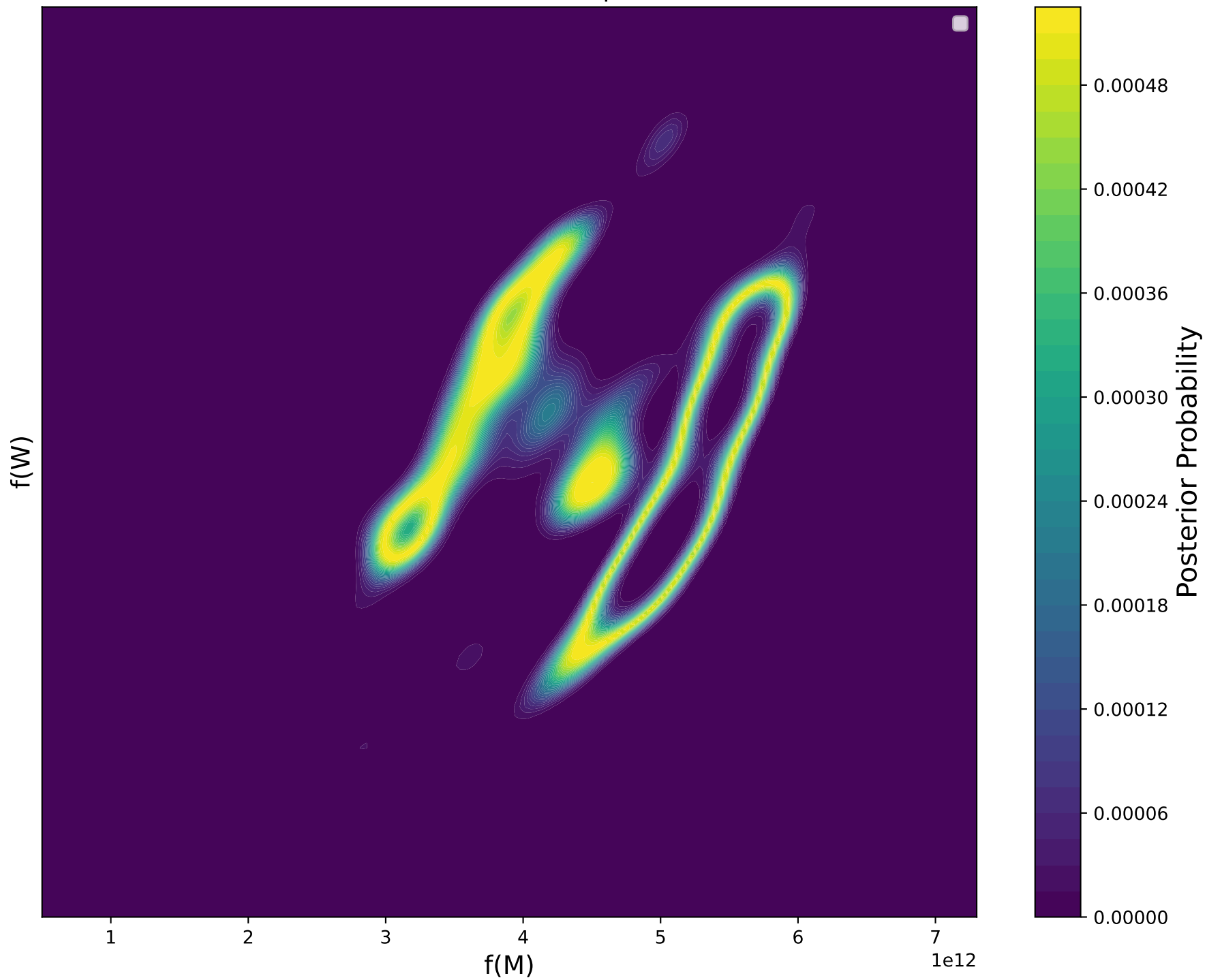
Posterior PDF, \pi(M, W|X = 11)
