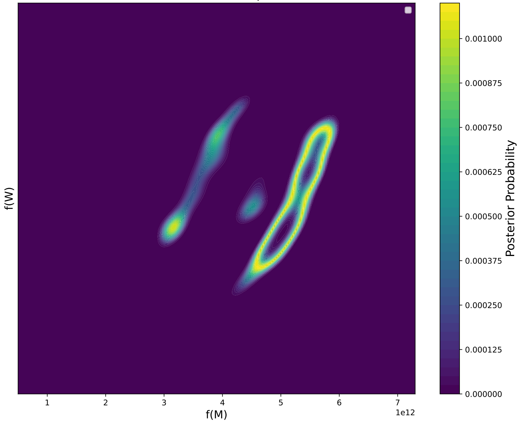
Posterior PDF, \pi(M, W|X = 16)
