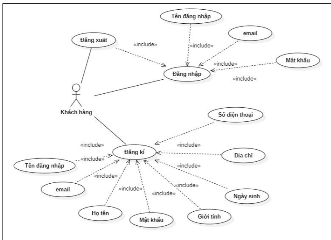
Hình số 9. Hình ảnh sơ đồ UseCase đăng kí và đăng nhập
