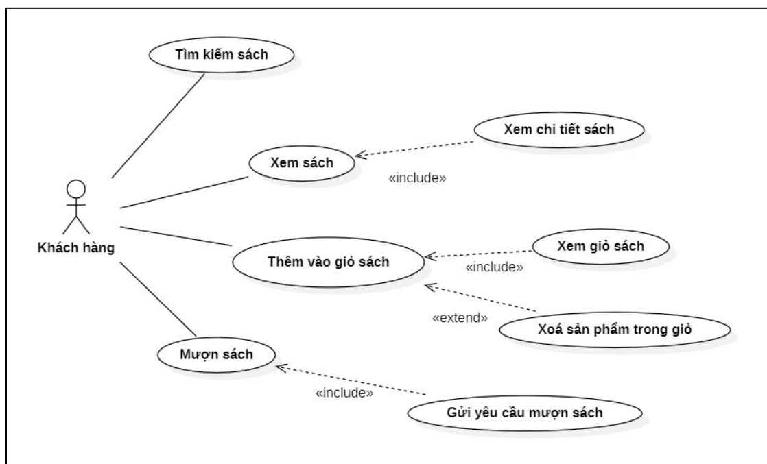
Hình số 10. Sơ đồ UseCase mượn sách
