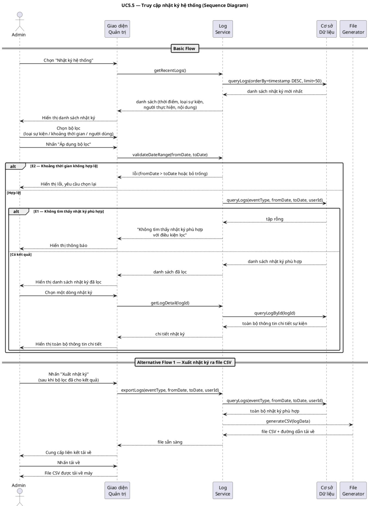
Hình 32: Sequence Diagram — UC5.5: Truy cập nhật ký hệ thống
