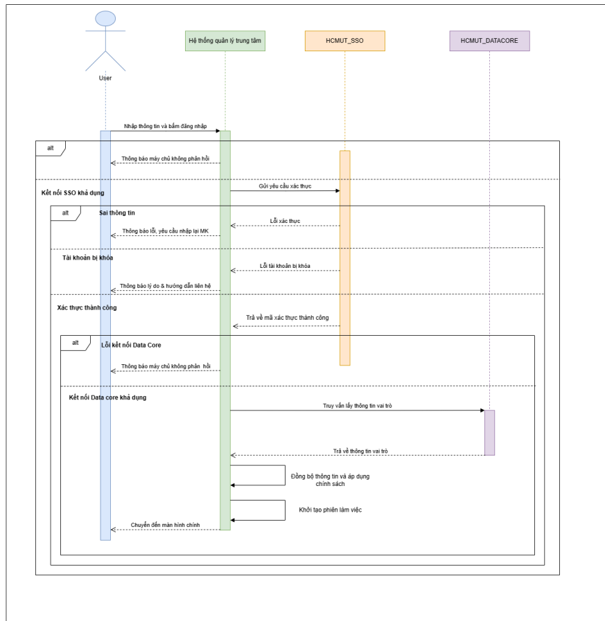
Hình 2: Sequence diagram cho Use-case U1.1: Đăng nhập vào hệ thống xác thực tập trung (SSO)
