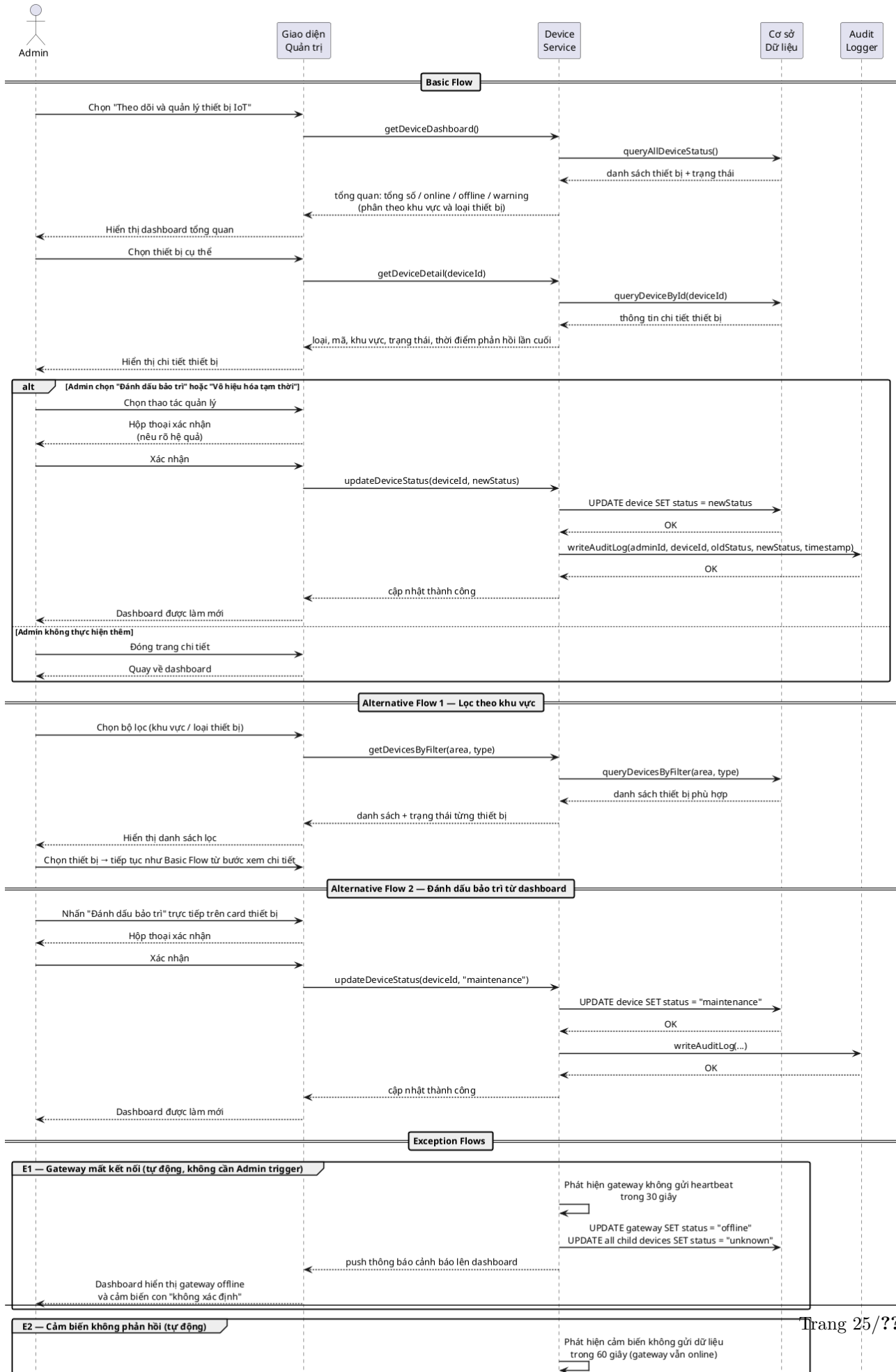
UC5.1 — Theo dõi và quản lý thiết bị IoT (Sequence Diagram)
