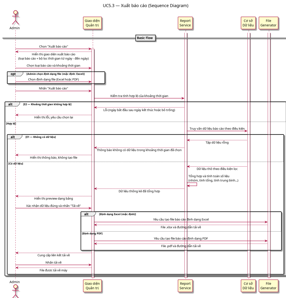
Hình 28: Sequence Diagram — UC5.3: Xuất báo cáo
