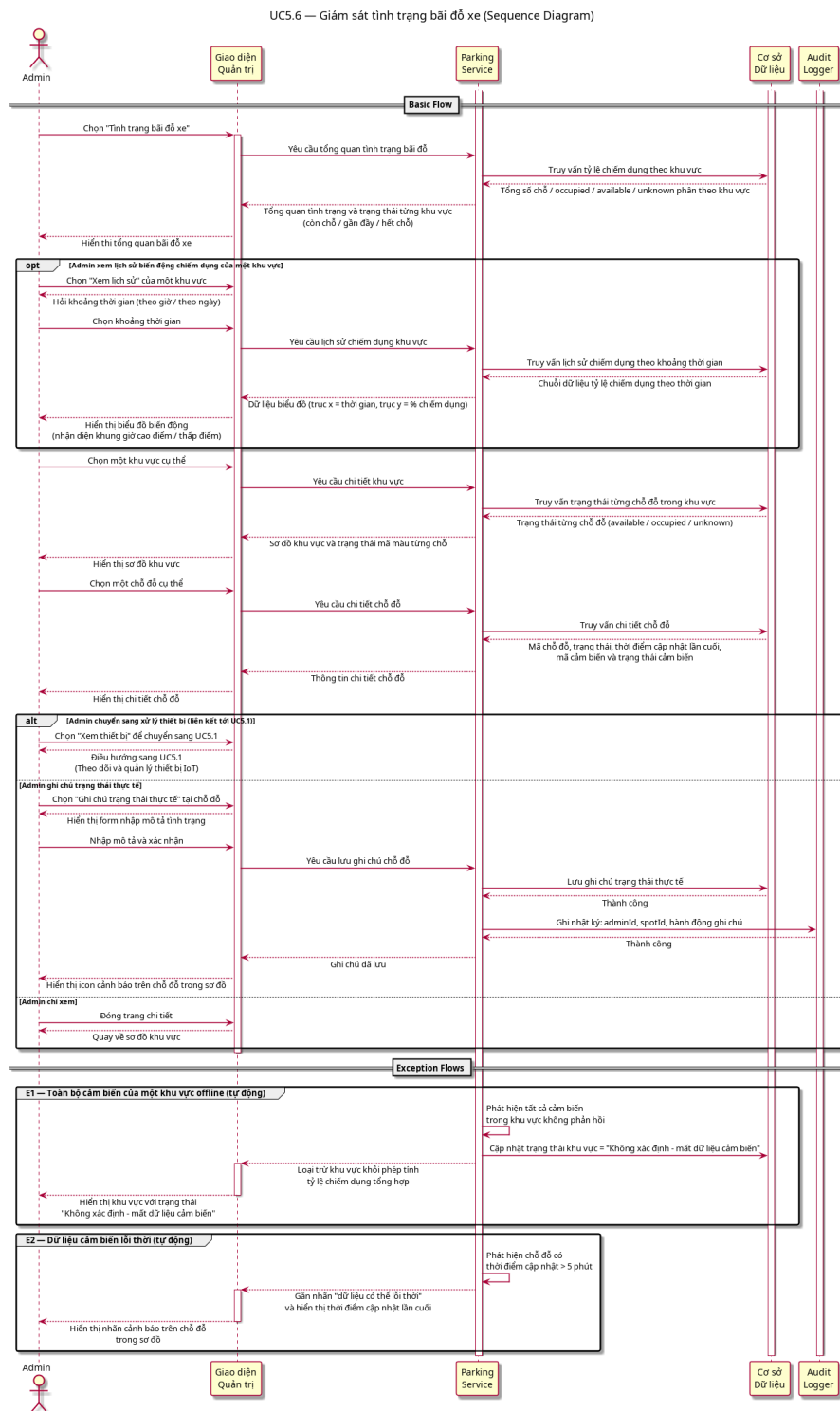
Hình 34: Sequence Diagram — UC5.6: Giám sát tình trạng bãi đỗ xe
