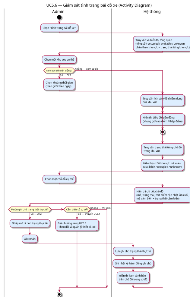
Hình 35: Activity Diagram — UC5.6: Giám sát tình trạng bãi đỗ xe
