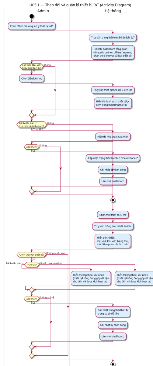
Hình 25: Activity Diagram — UC5.1: Theo dõi và quản lý thiết bị IoT
