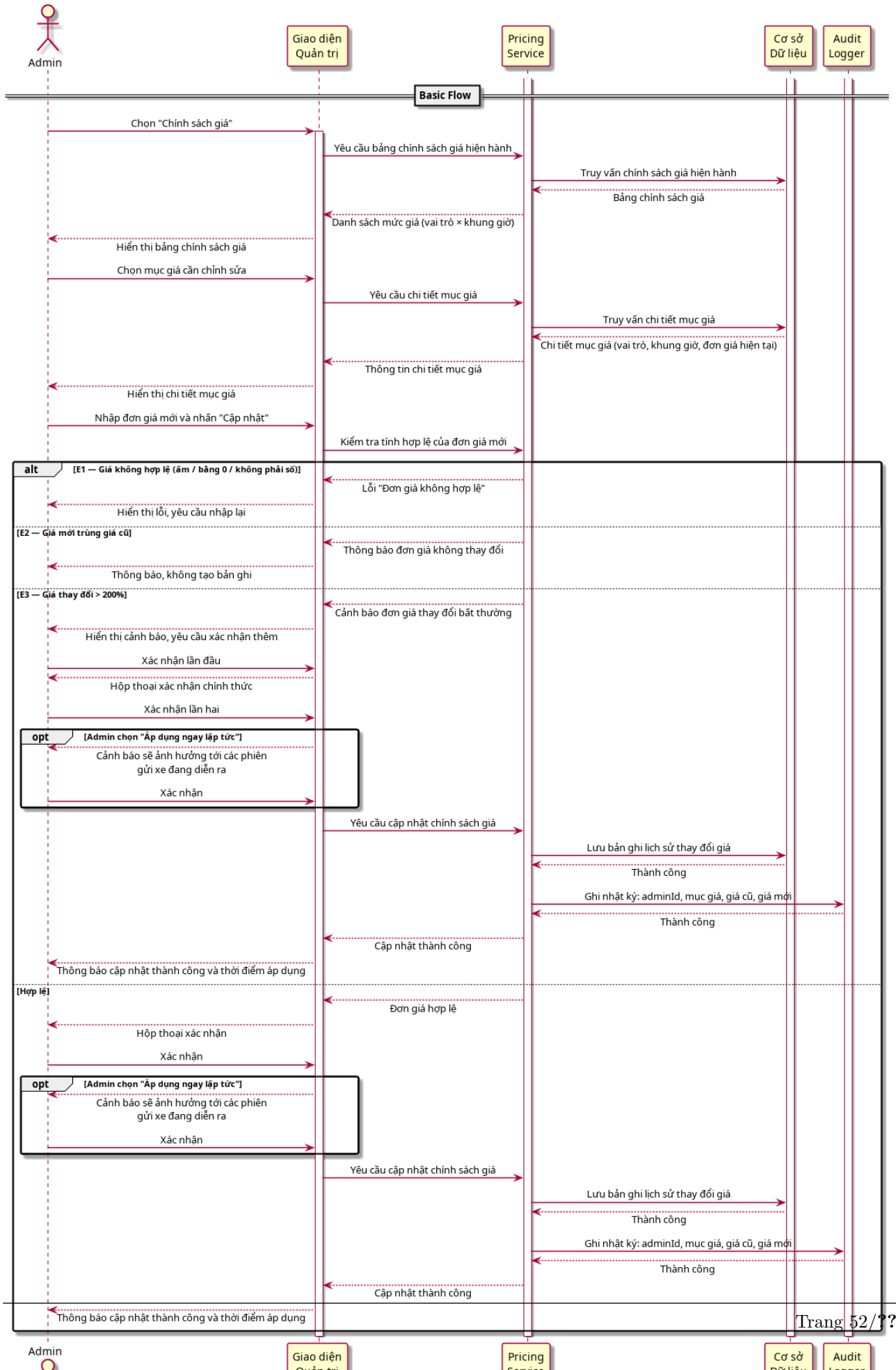
UC5.4 — Thay đổi chính sách giá (Sequence Diagram)
