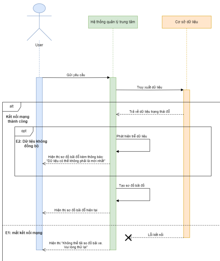
Hình 20: Sequence Diagram — U4.2: Hiện thị trạng thái bãi xe
