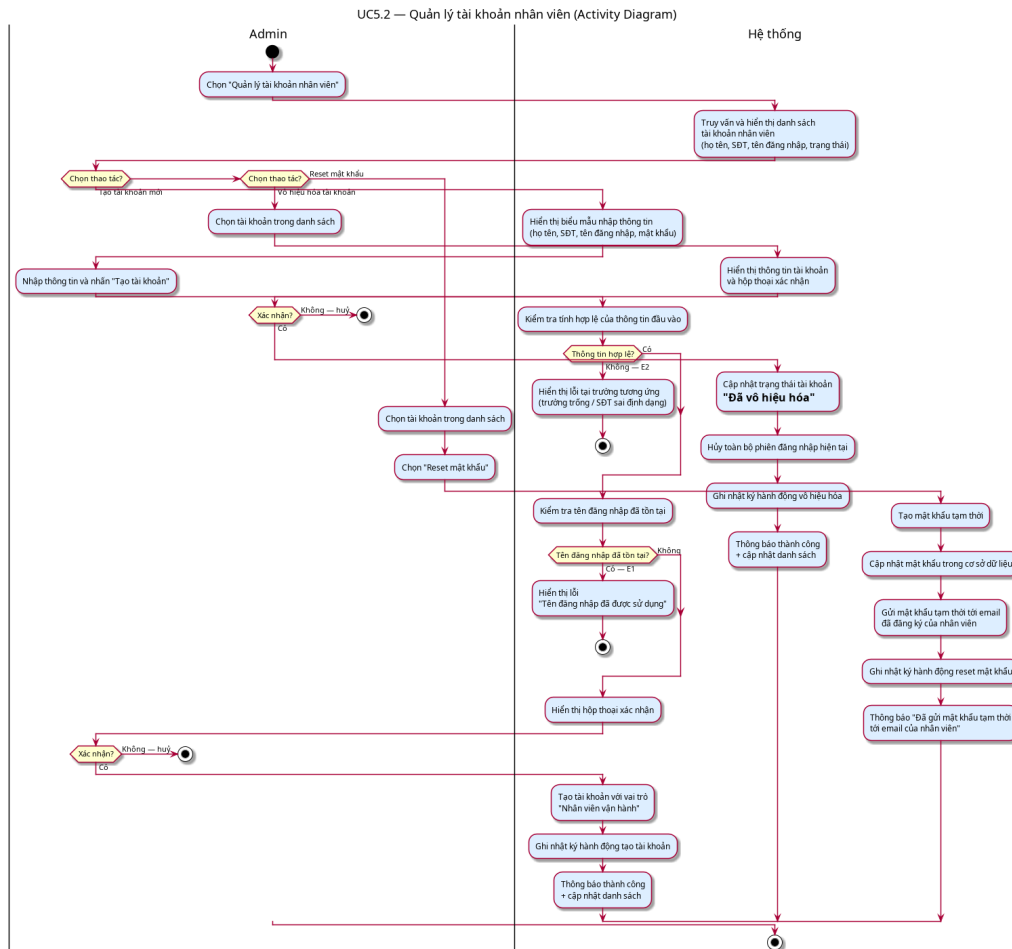
Hình 27: Activity Diagram — UC5.2: Quản lý tài khoản nhân viên
