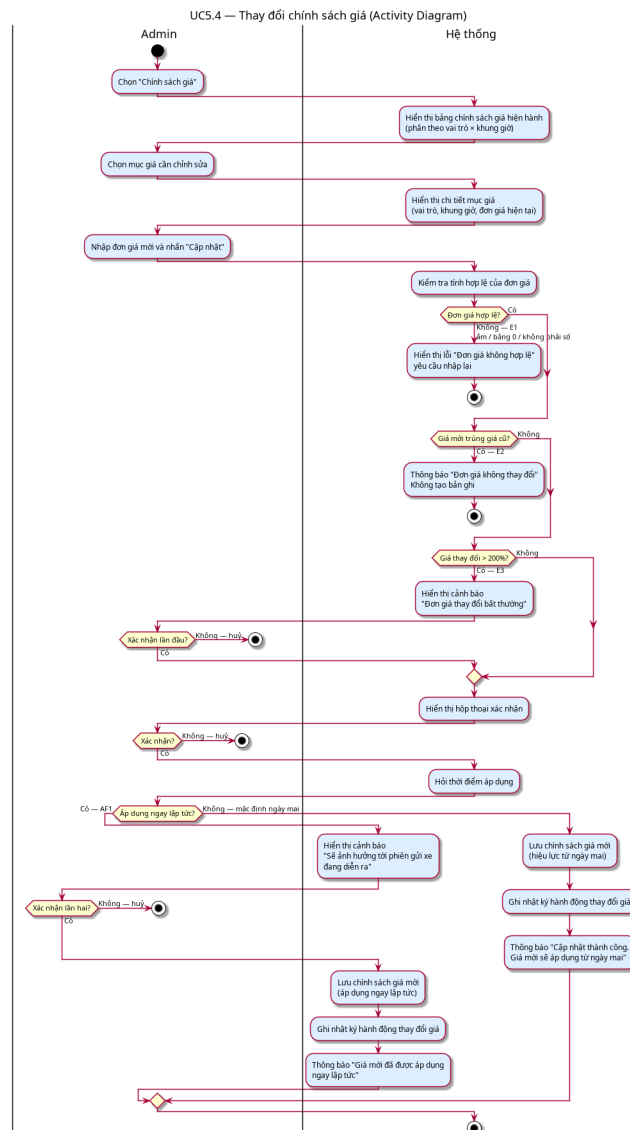
Hình 31: Activity Diagram — UC5.4: Thay đổi chính sách giá
