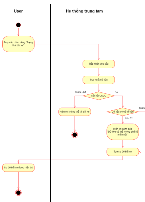
Hình 21: Activity Diagram — U4.2: Hiện thị trạng thái bãi xe
