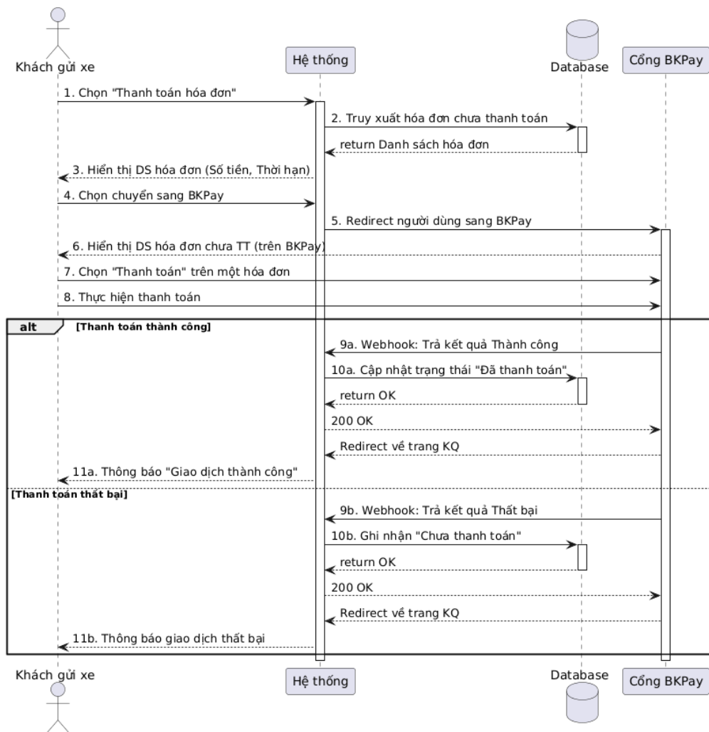
Hình 6: Sequence diagram cho Use-case U3.2: Thanh toán hóa đơn
