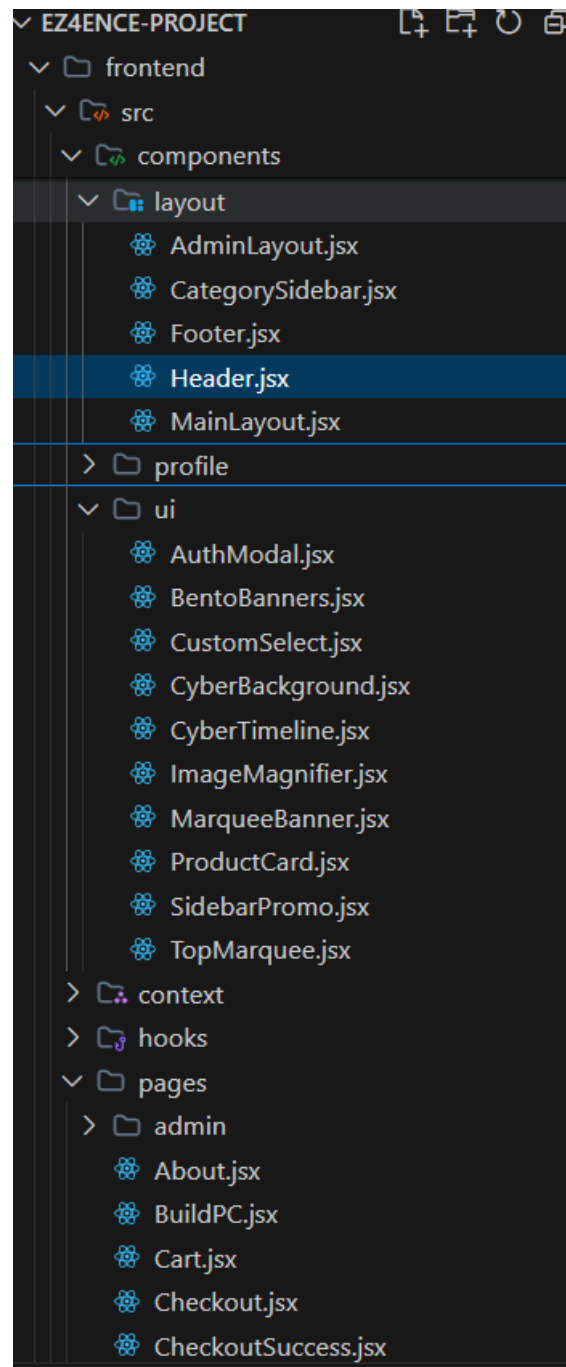
Hình 3: Cấu trúc source chứa Header, Footer, Banner.
