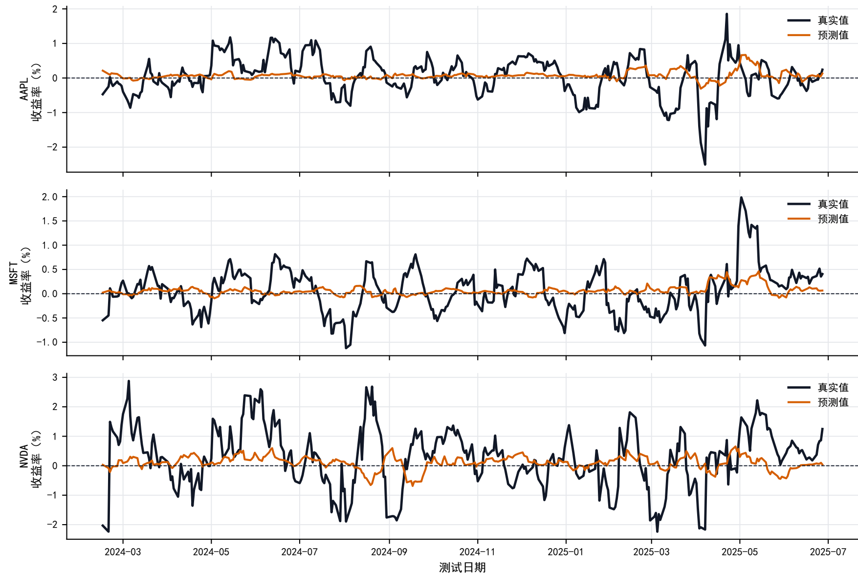
单只股票真实收益与预测收益曲线 (P-sLSTM-DA Focal)
