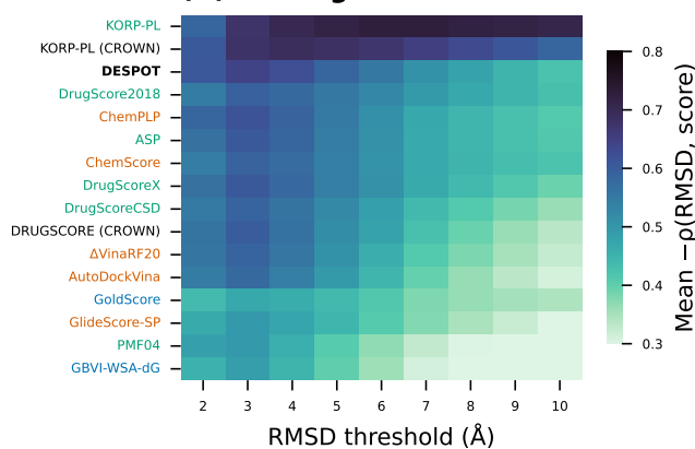
(D) Binding funnel
