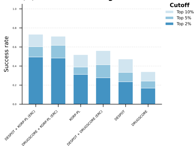
(D) Reverse screening
