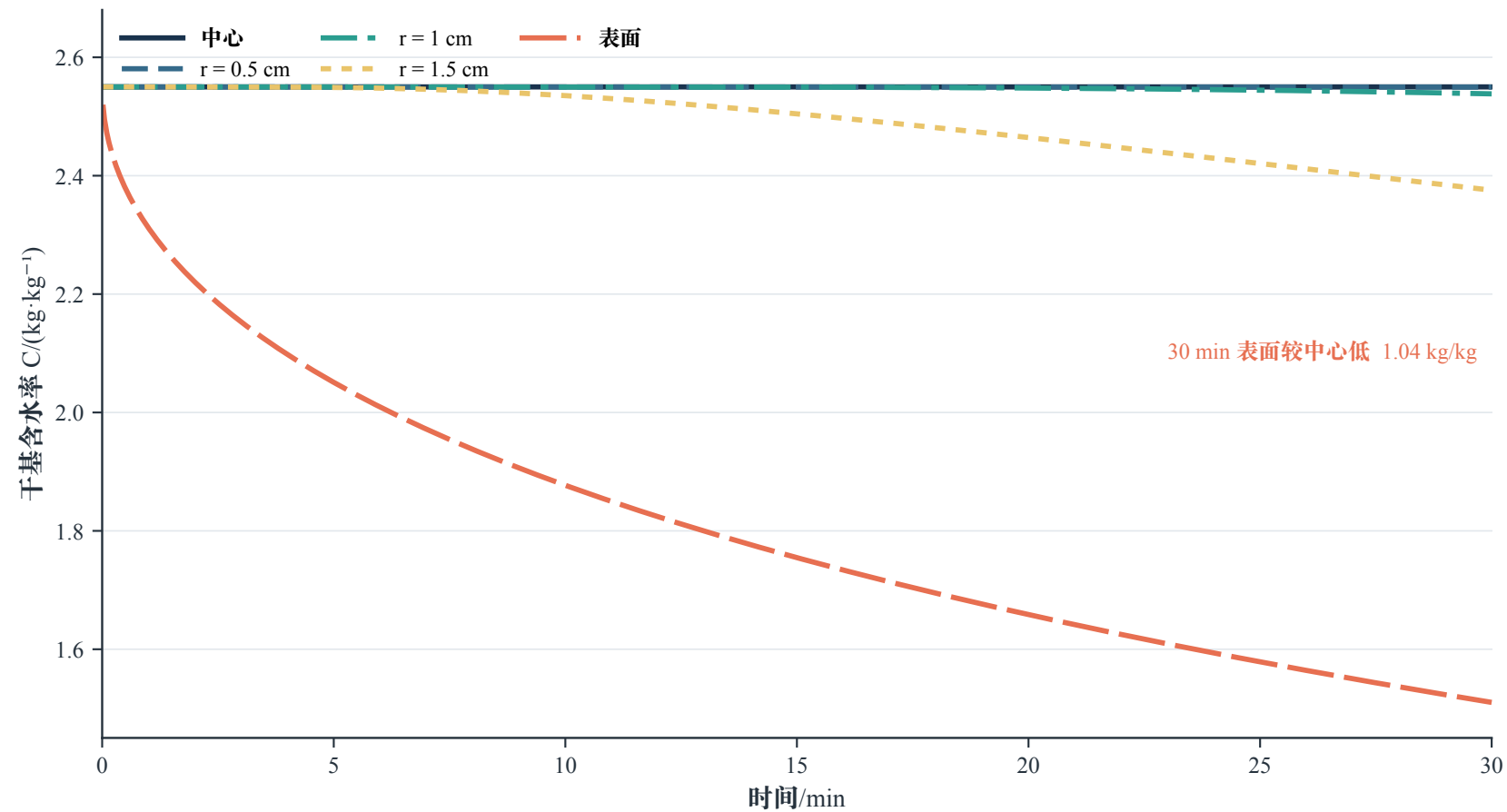
径向各位置的含水率演化
