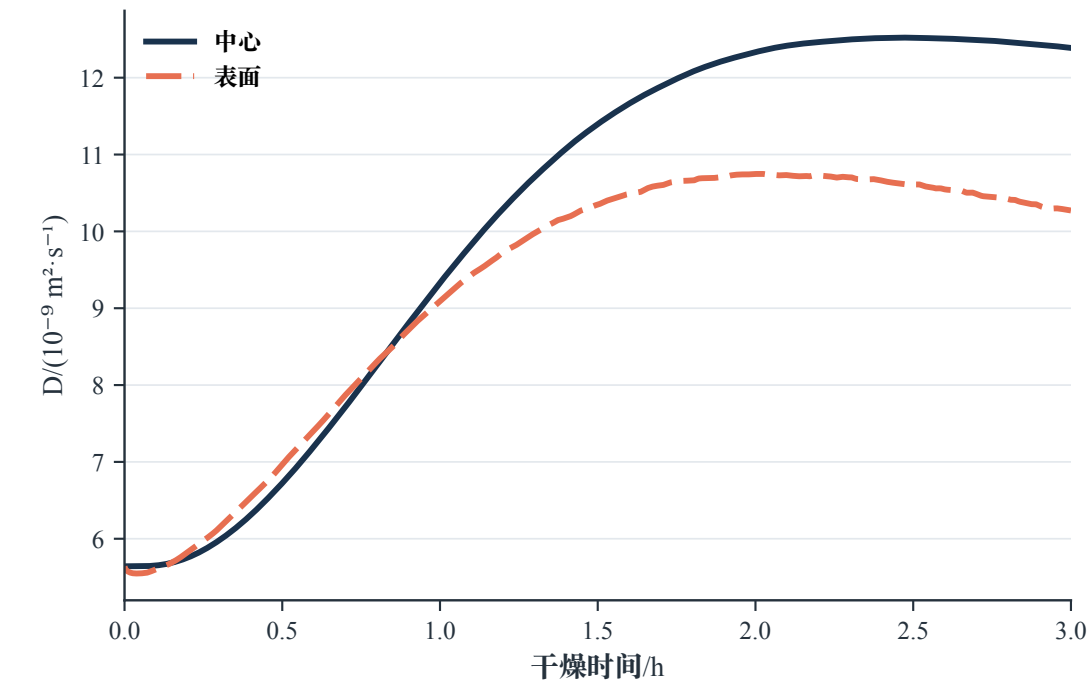
有效水分扩散系数
