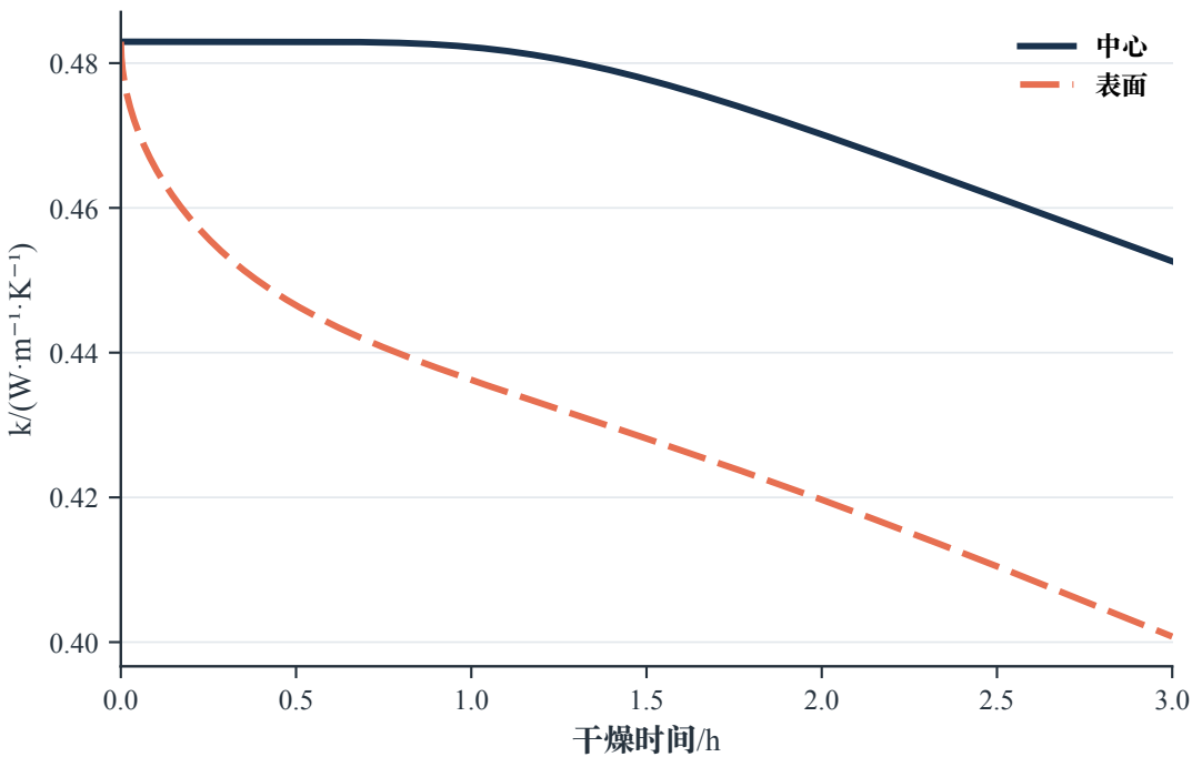
导热系数
