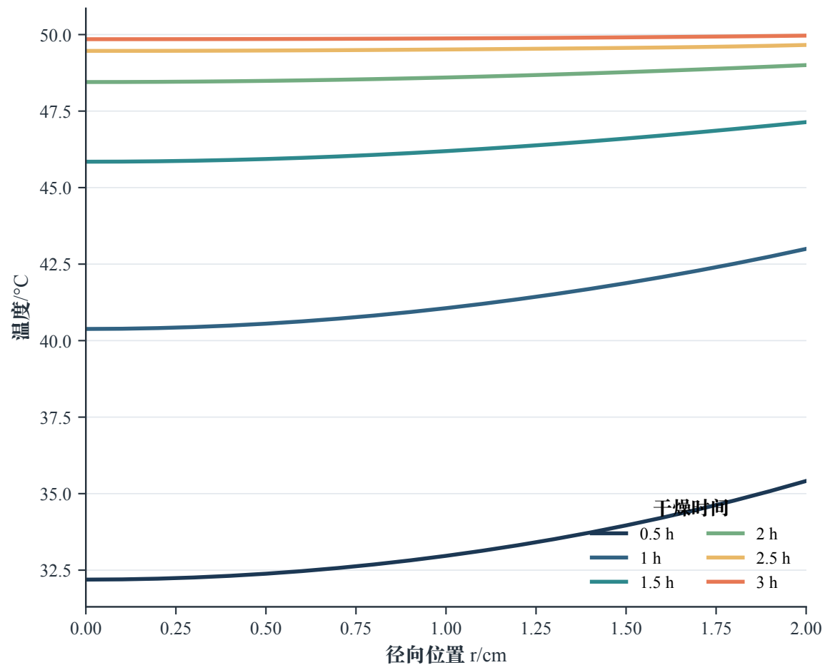
温度径向剖面
