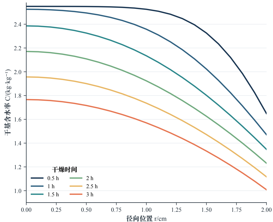
含水率径向剖面
