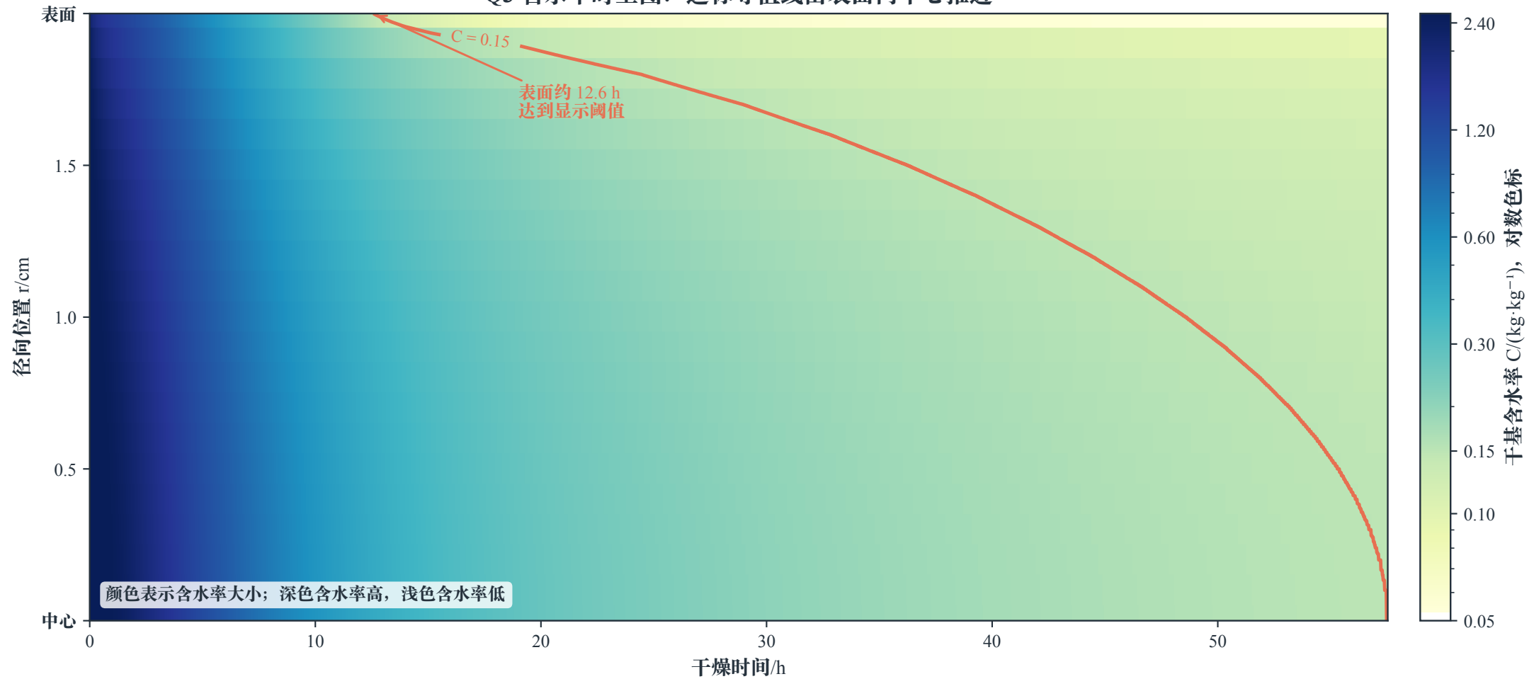
Q3 含水率时空图：达标等值线由表面向中心推进
