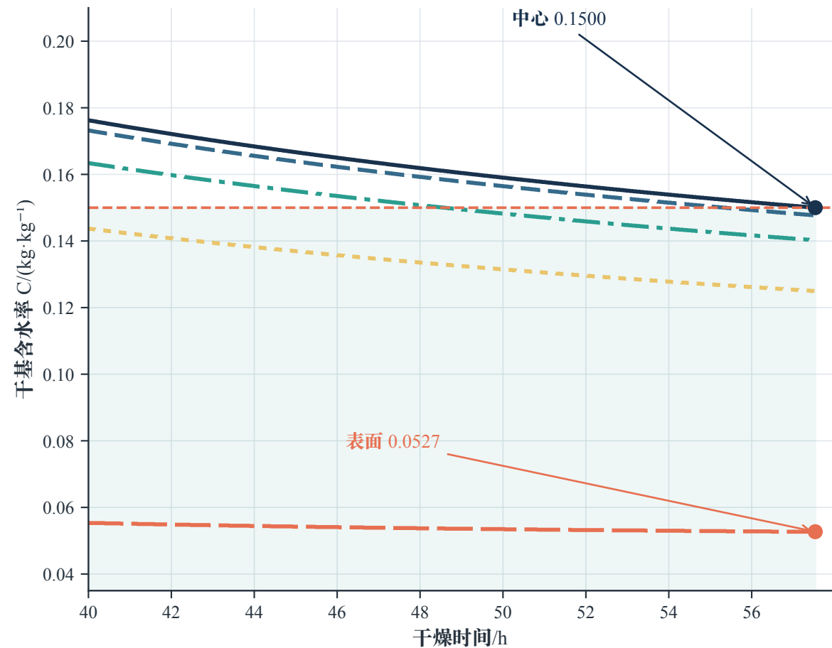
末段放大：中心控制终止时刻
