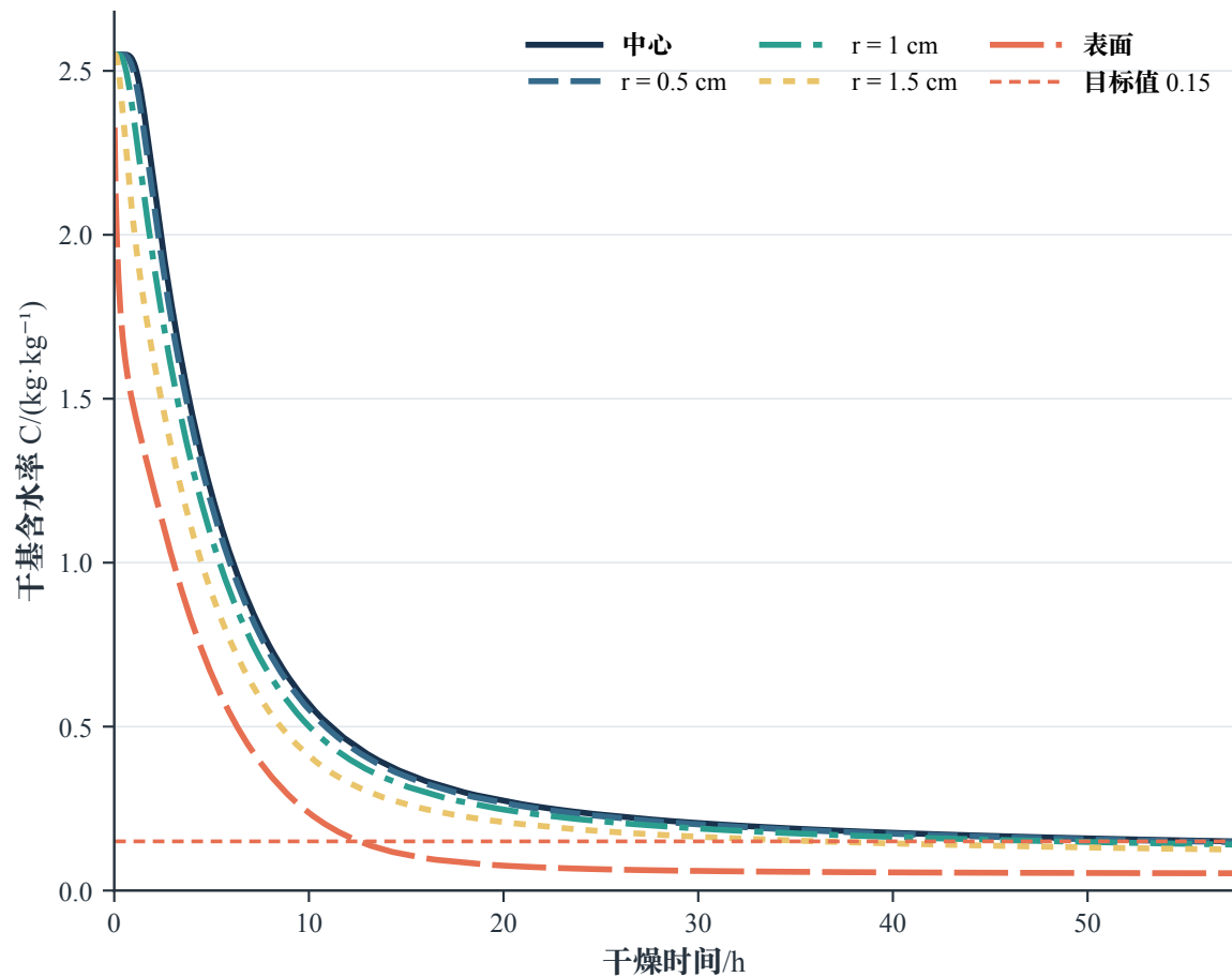
全程响应：表面先干，中心后达标
