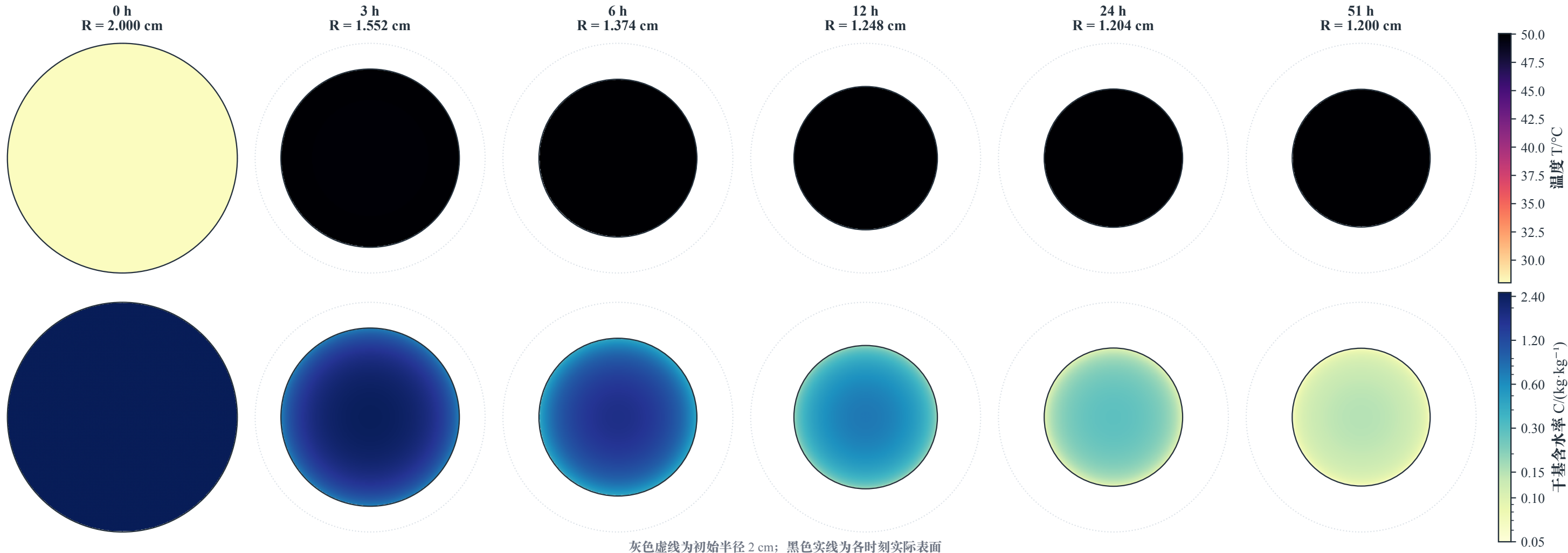
Q4 真实尺寸圆截面演化：颜色变化与几何收缩同步可见
