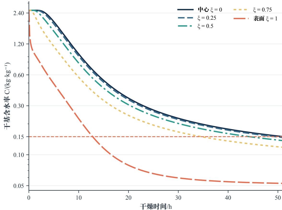
材料层含水率响应
