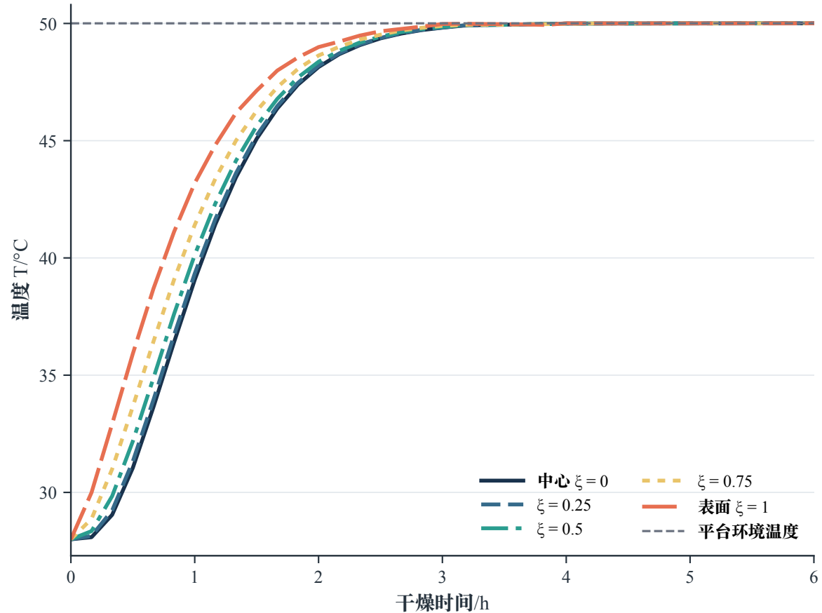
材料层温度响应 (前 6 h 放大)
