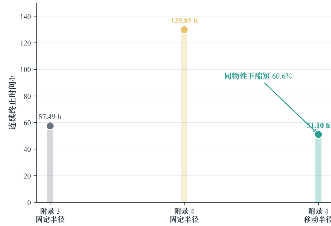
三组同离散模型拆分物性与收缩效应
