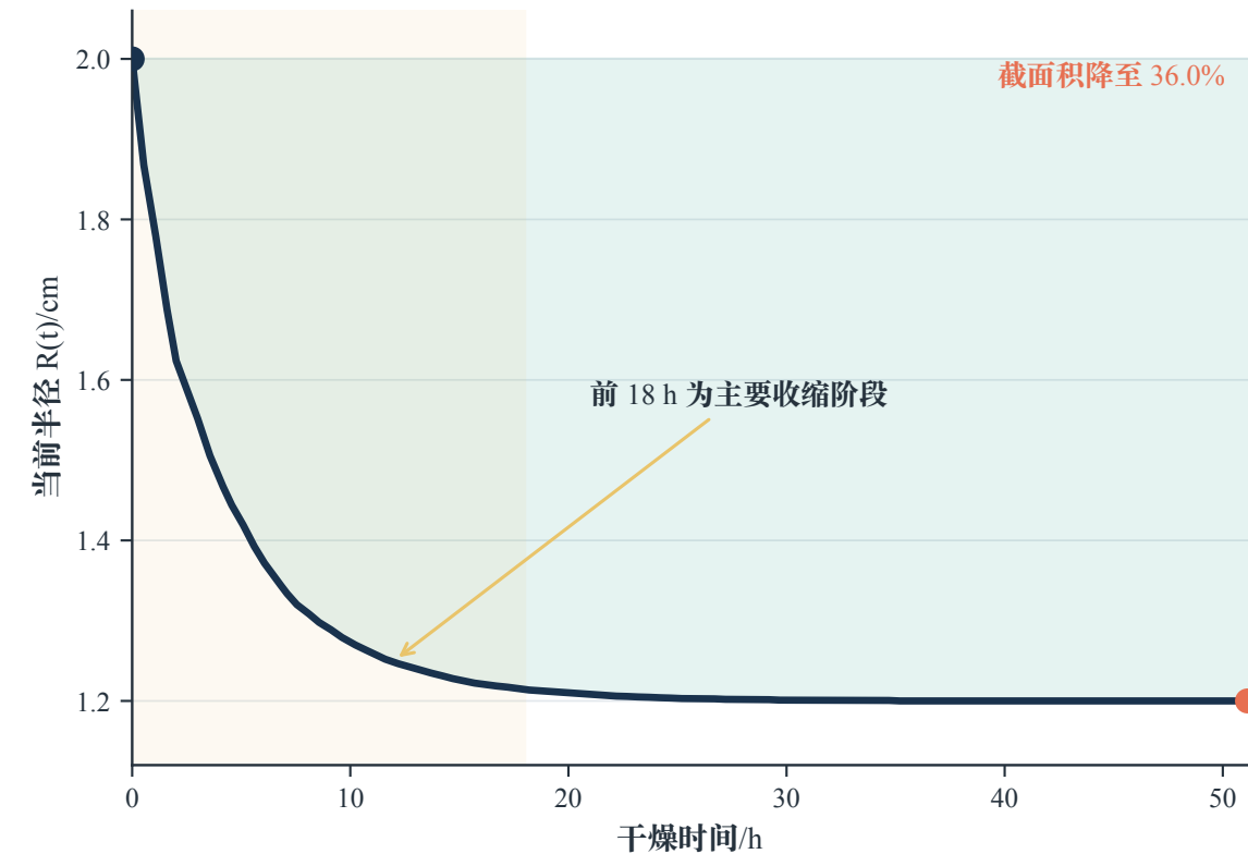
给定半径历史
