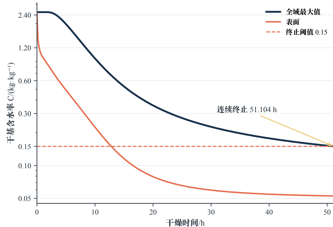
中心控制最终达标
