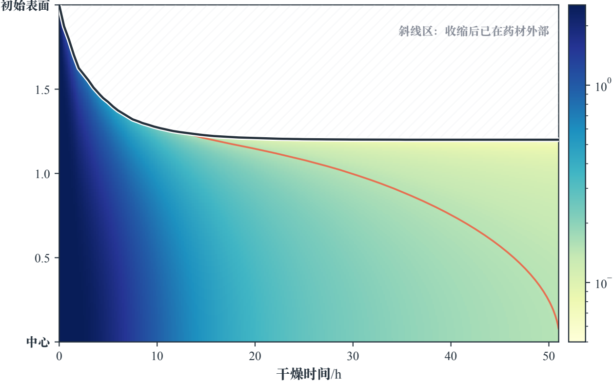
物理域含水率：边界以内才有材料
