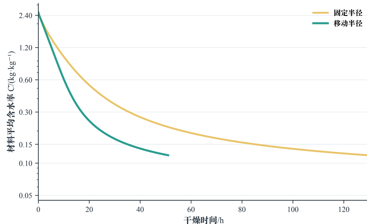
烘干时长分解
