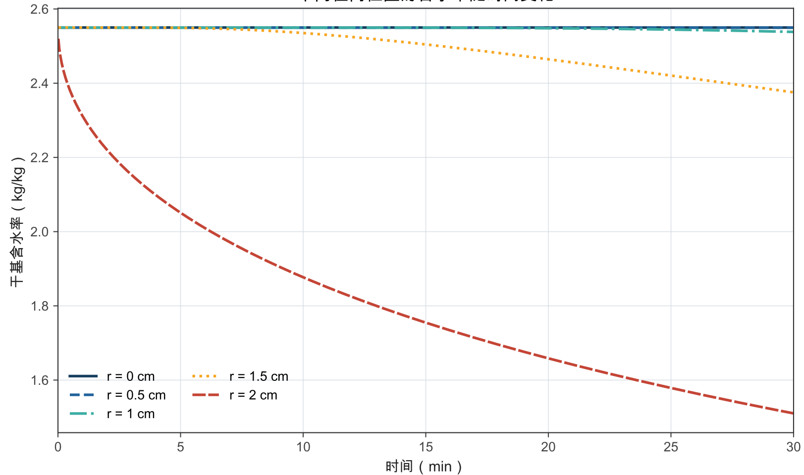
不同径向位置的含水率随时间变化
