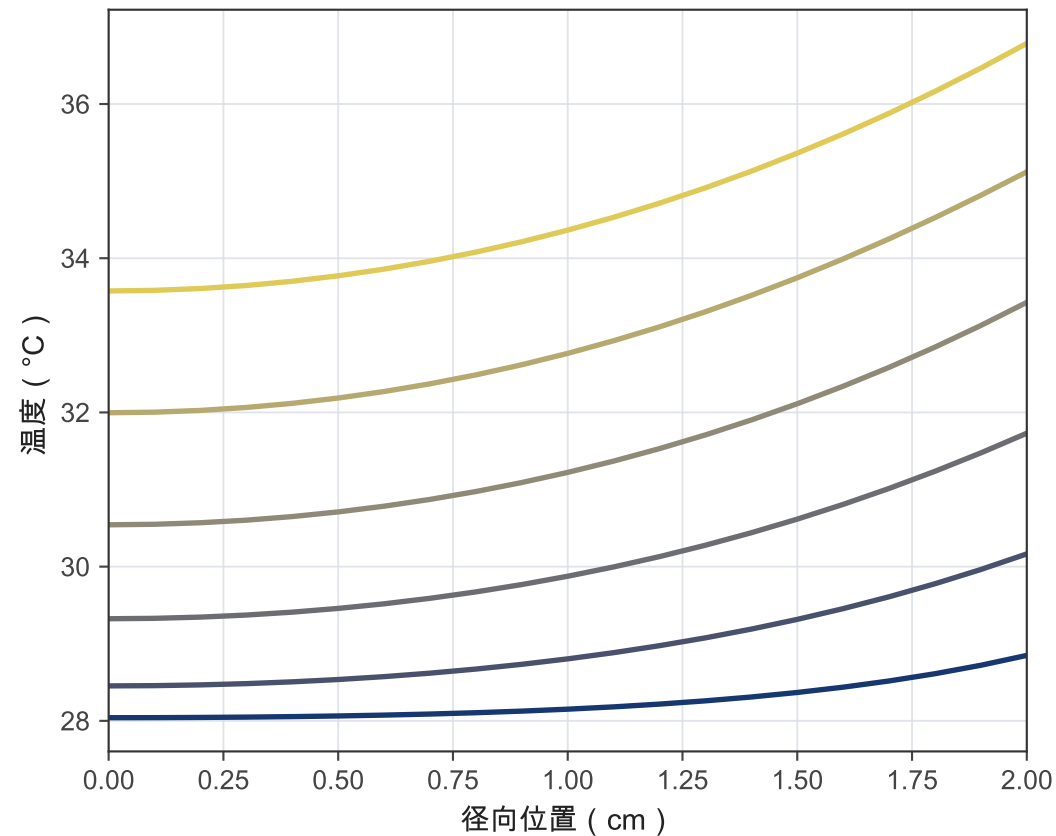
不同时刻的径向温度剖面
