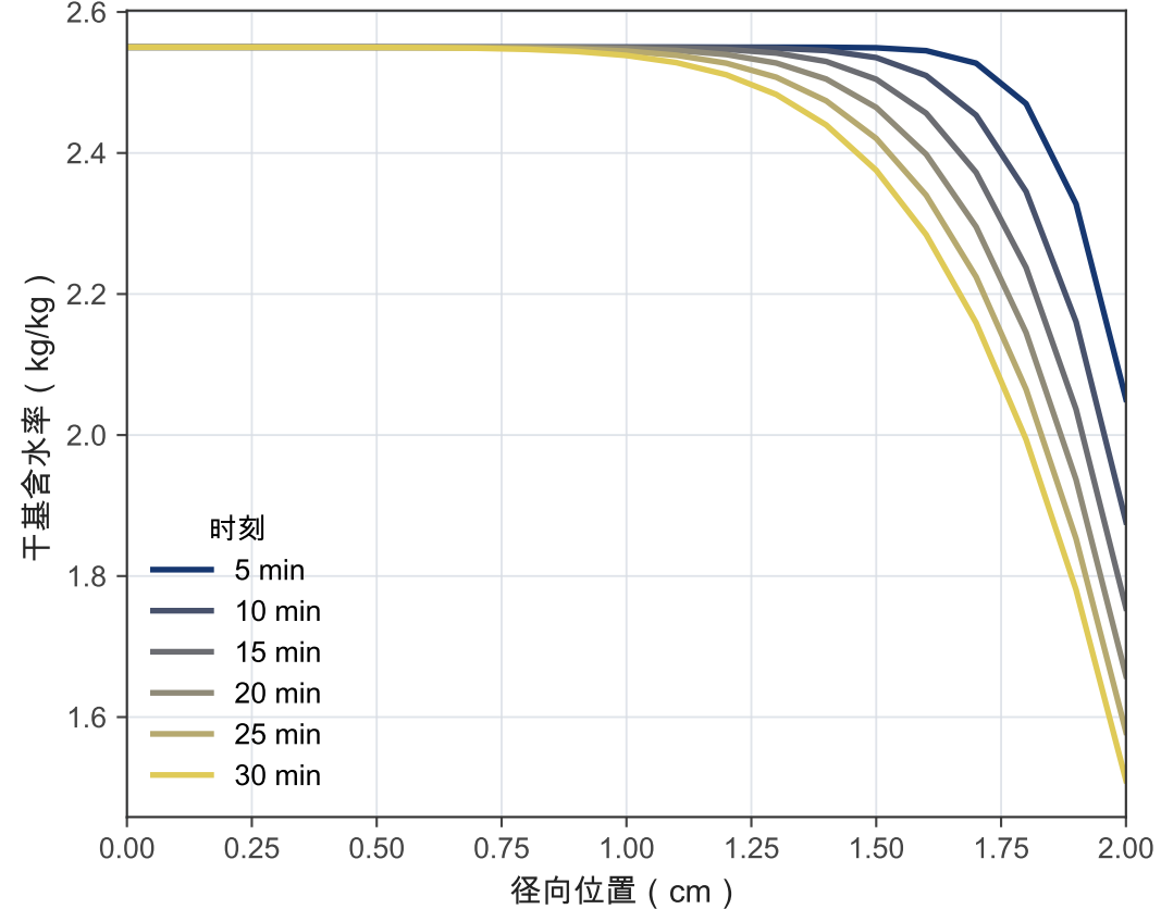
不同时刻的径向含水率剖面
